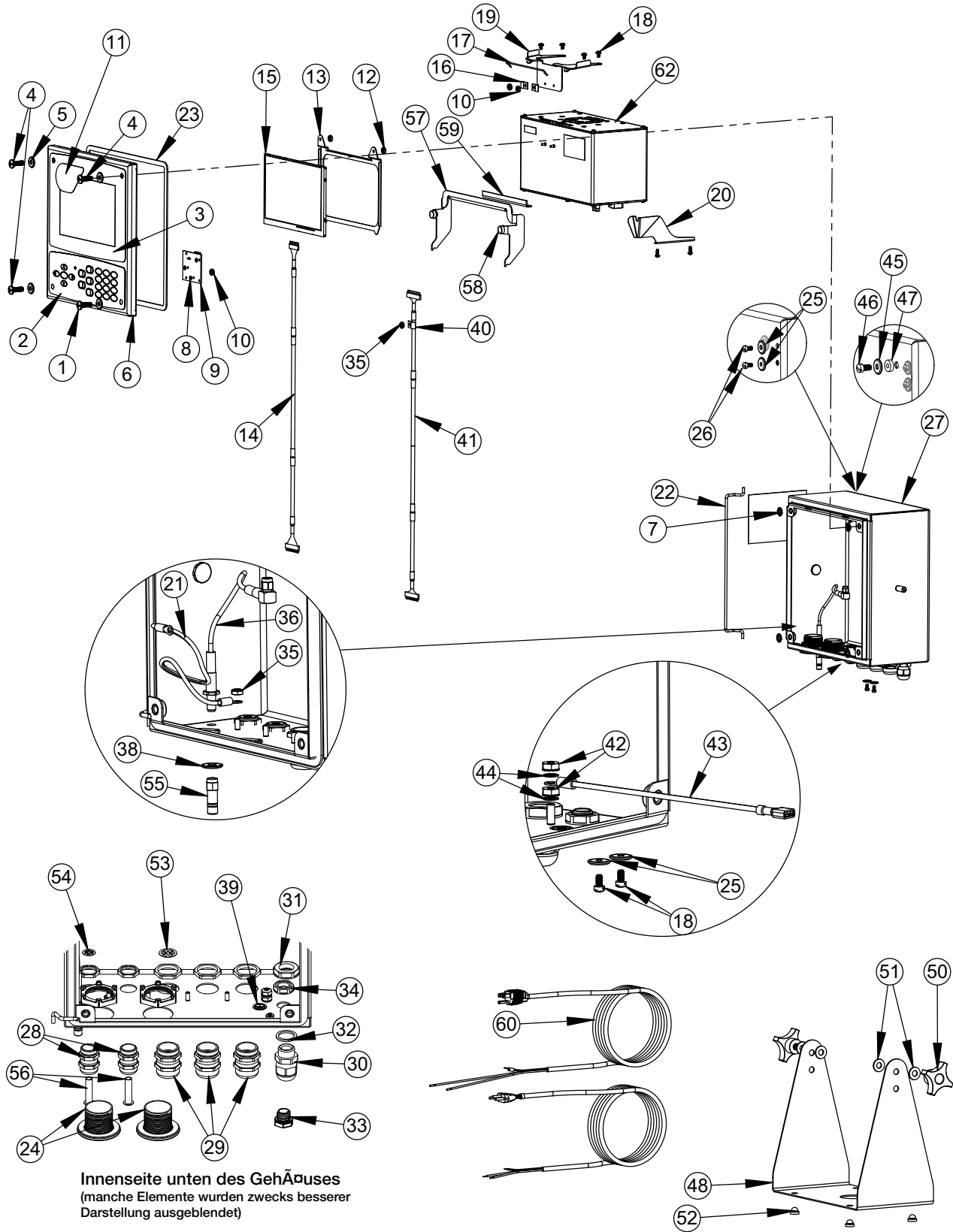
Abbildung 2-40. UniversalgehÄuse - Reparaturteile
