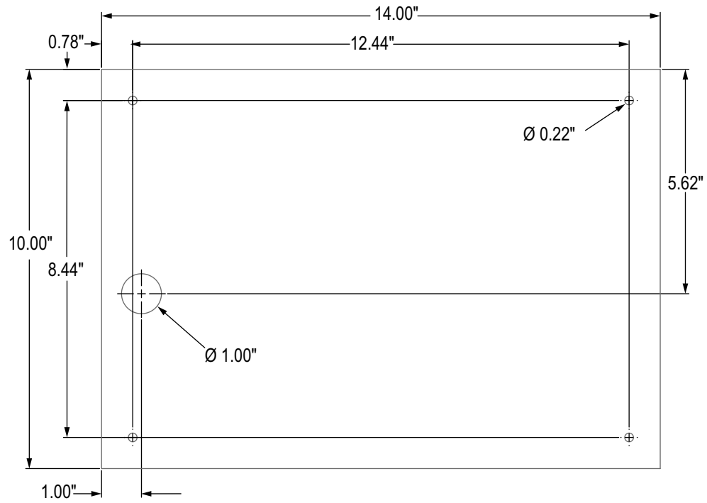
Abbildung 2-17. Abmessungen für die 12"-Schalttafel (nur Touch)
