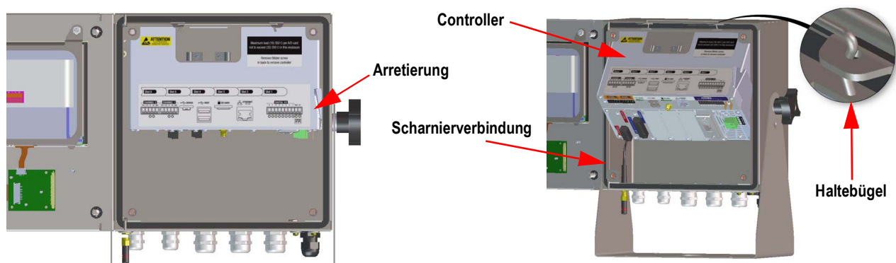
Abbildung 2-4. Entfernen der CPU - Universalhalterung
