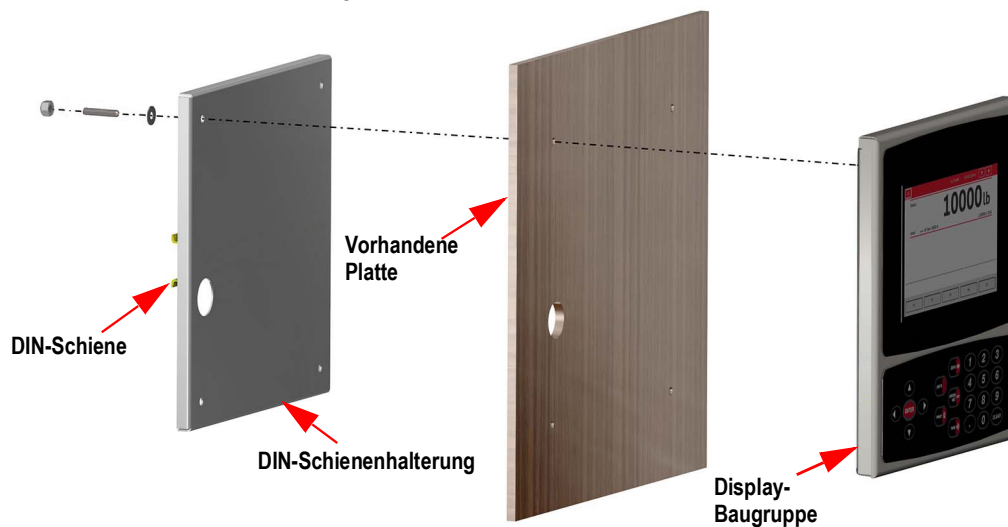
Abbildung 2-14. Schalttafeleinbau
