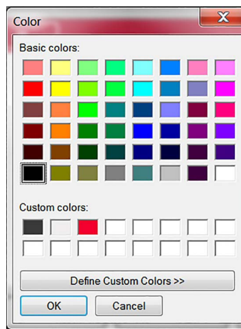
Abbildung 14-15. Widget-Farben
