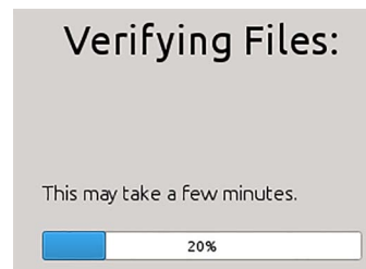
Abbildung 13-11. Dateiprüfung
