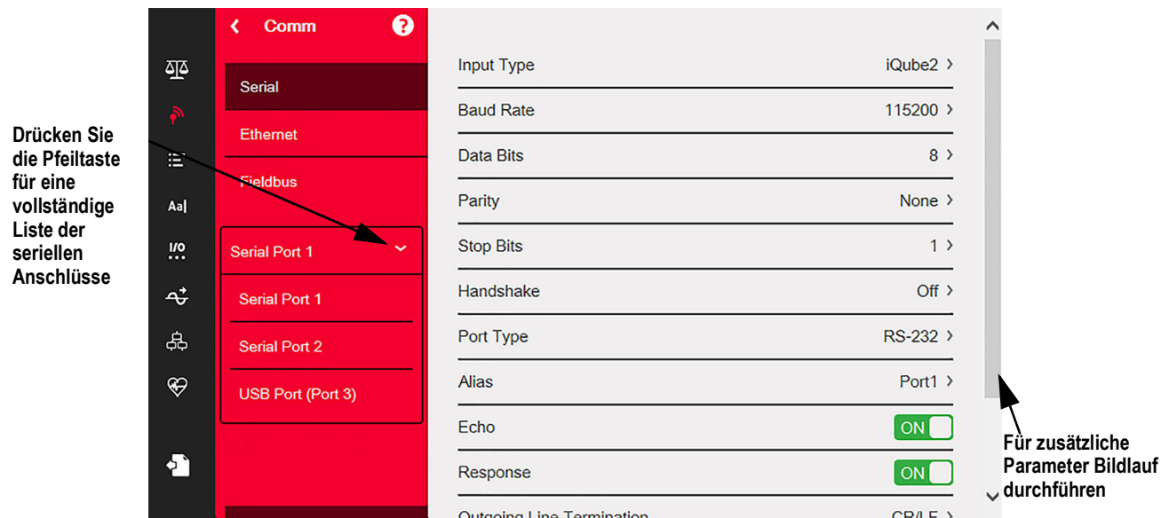
Abbildung 5-2. Menü „Serial“
