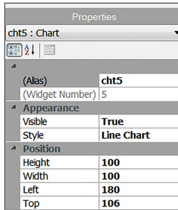
Abbildung 14-12. Chart Widgets
