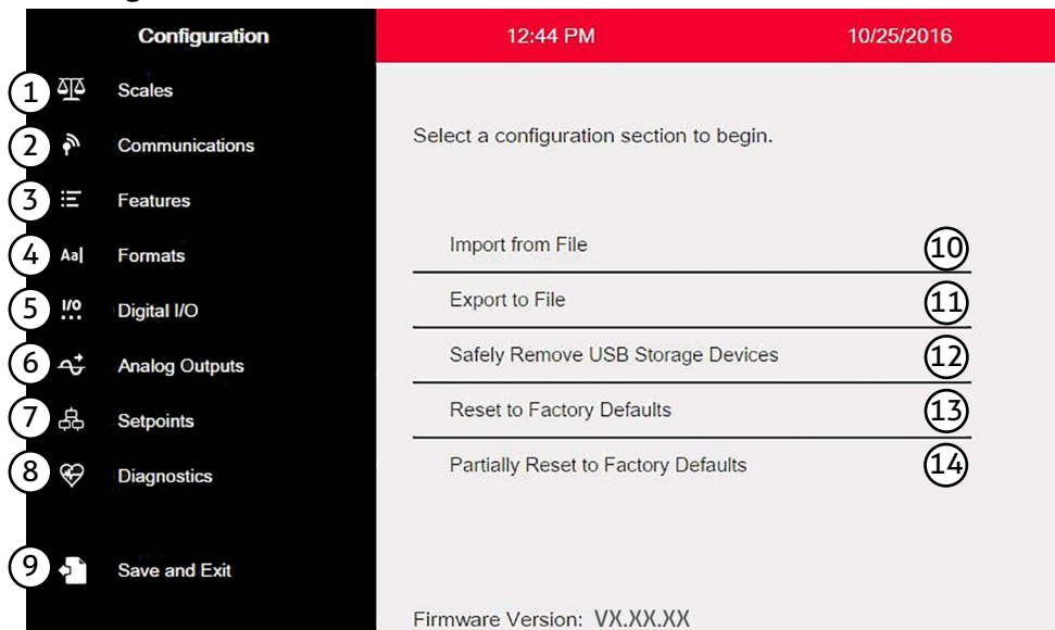
Abbildung 3-4. Menü „Configuration“
