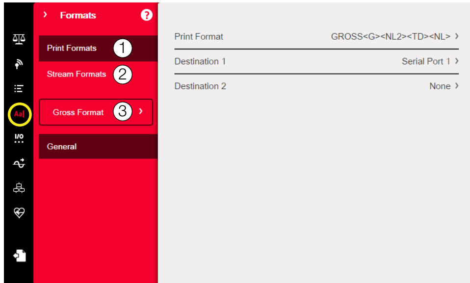
Abbildung 7-1. Menü „Format“
