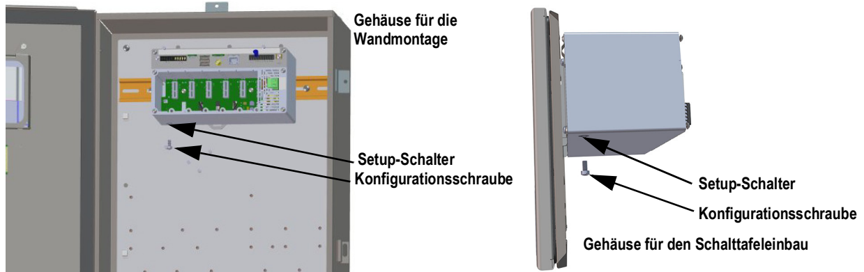
Abbildung 3-2. Positionen des Setup-Schalters (Gehäuse für Schalttafel-/Wandmontage)
