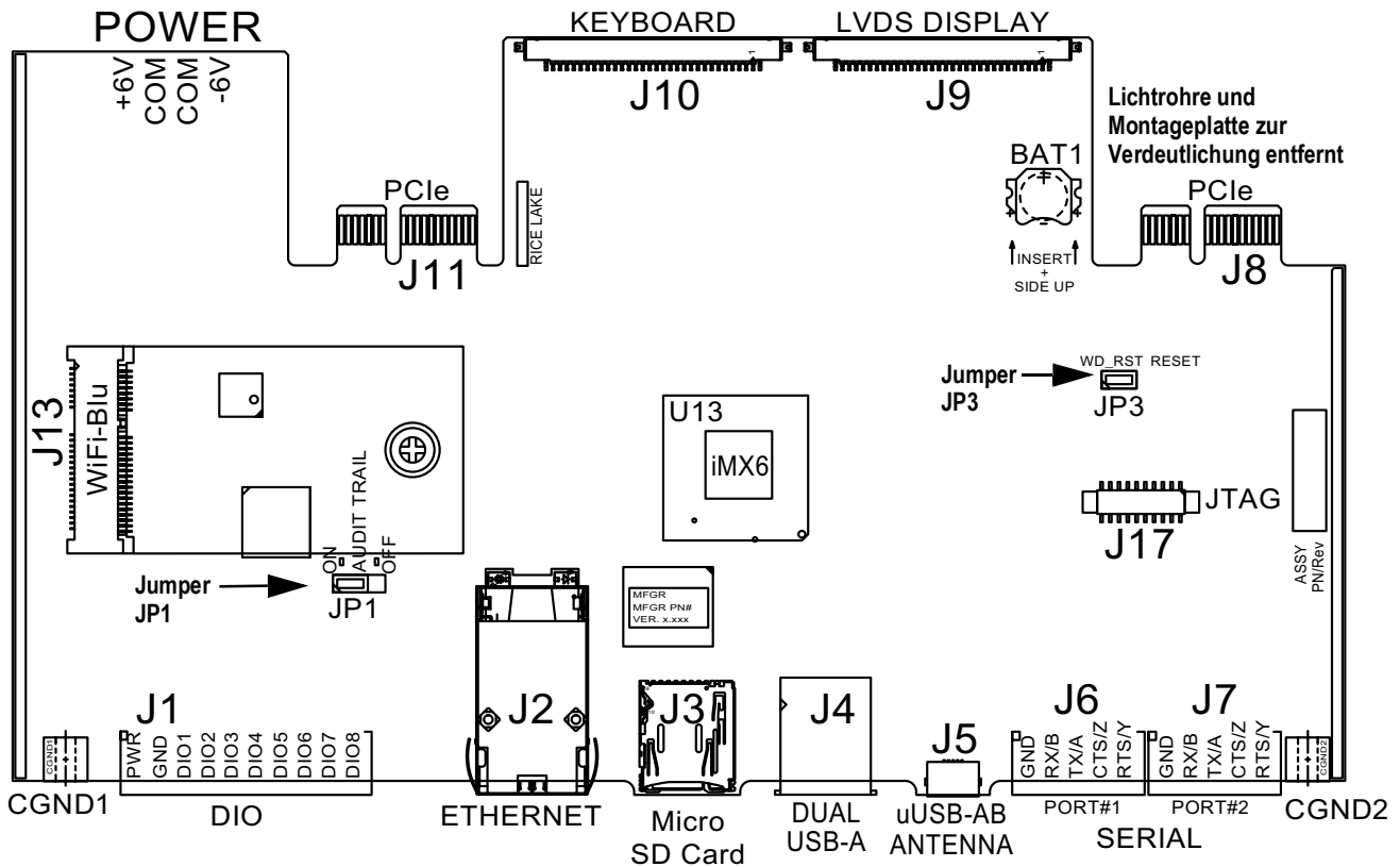
Abbildung 3-3. Jumper-Positionen
