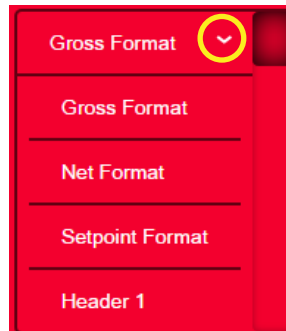
Abbildung 7-2. Formatauswahl
