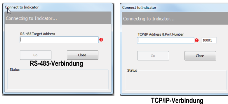
Abbildung 13-7. Verbindungsbildschirme
