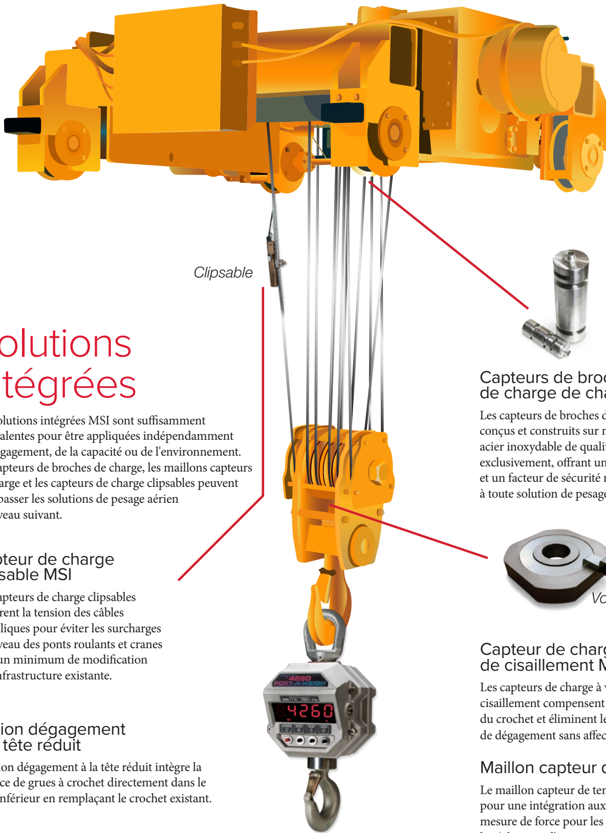
Balances de grue
