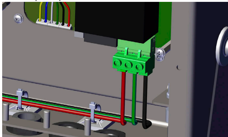
Illustration 2-22. Branchement du câble d'alimentation en courant continu
