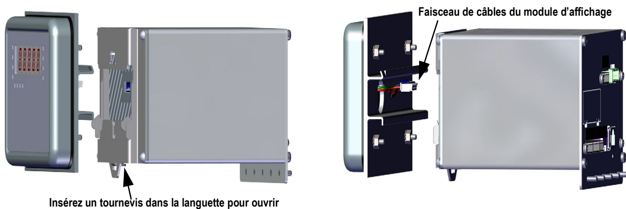
Illustration 2-4. Installation du contrôleur
