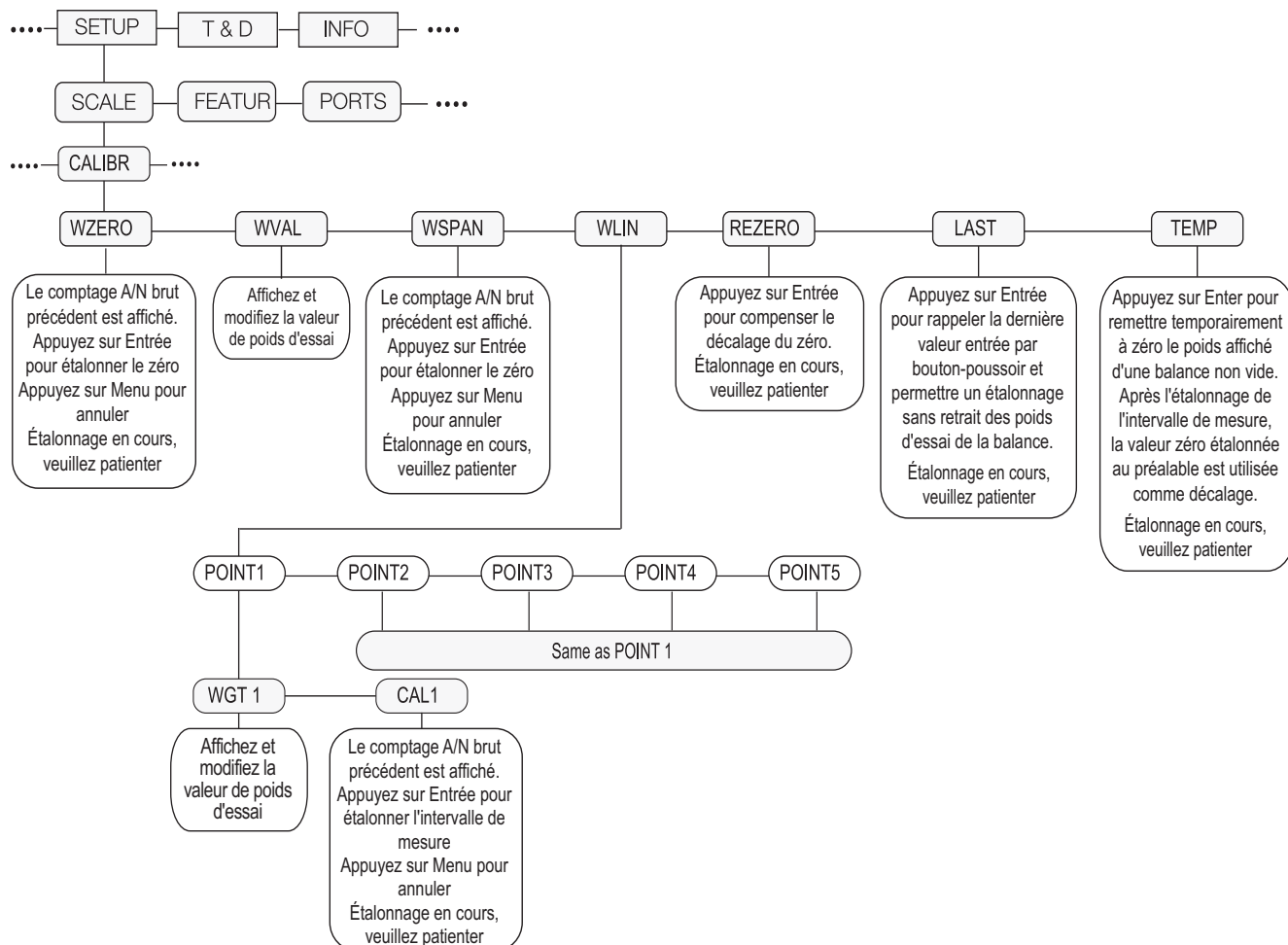
Illustration 3-8. Structure du menu d'étalonnage
