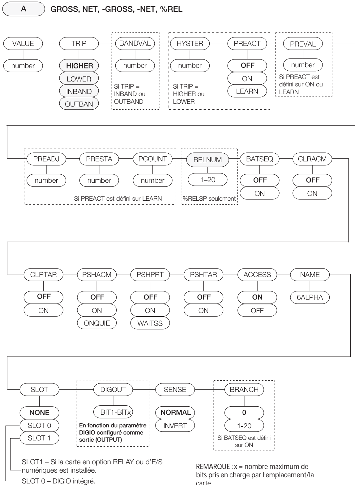
Illustration 3-18. Structure du menu de points de consigne – Structure A
