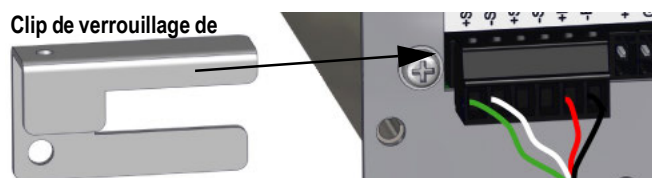
Illustration 2-26. Installation du clip de verrouillage de capteur de charge
