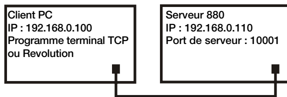
Illustration 9-1. Connexion directe de l'ordinateur au serveur Ethernet de l'indicateur 880
