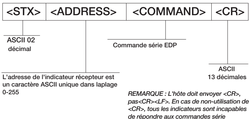
Illustration 10-2. Format de données pour les envois RS-485
