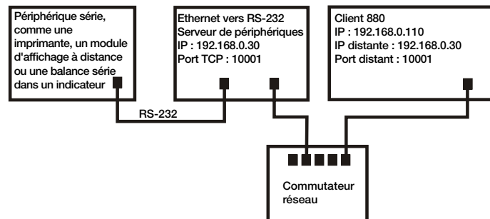
Illustration 9-4. Envoi ou demande de données à un serveur distant de périphériques Ethernet - RS232
