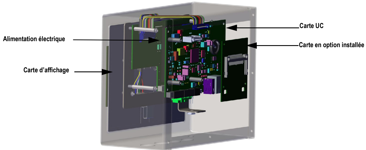
Illustration 2-15. Emplacements des cartes dans le boîtier universel
