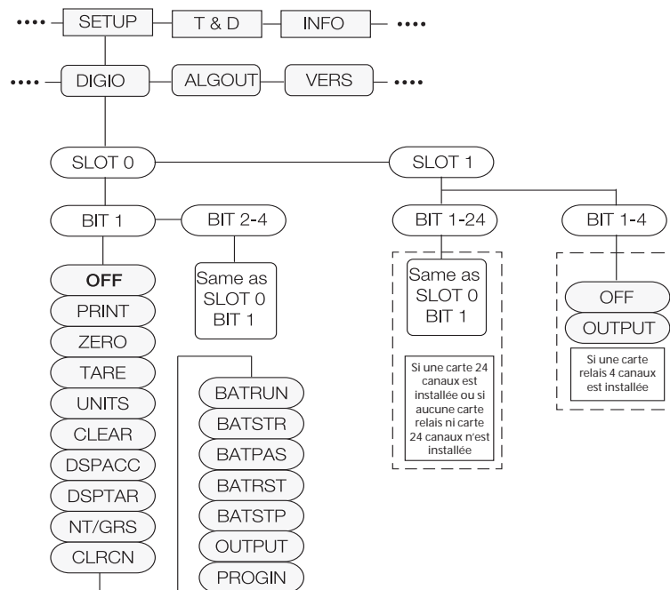
Illustration 3-22. Menu d'E/S numériques
