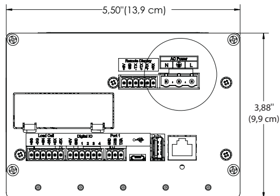
Illustration 2-1. Dimensions de l'indicateur 880 à boîtier pour installation à panneau
