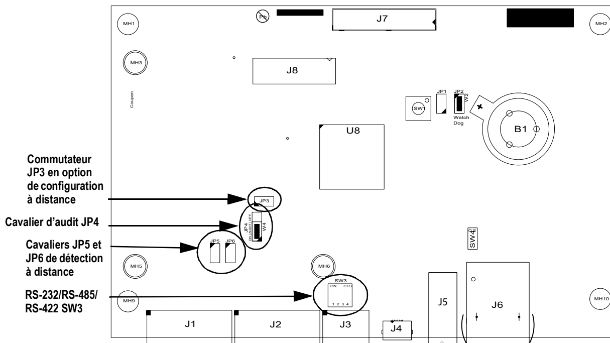
Illustration 2-24. Carte UC d'indicateur 880
