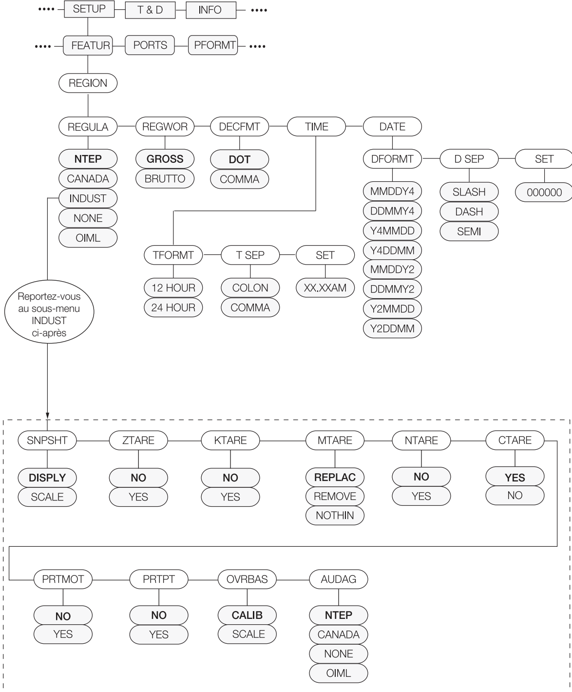
Illustration 3-10. Structure du menu Région
