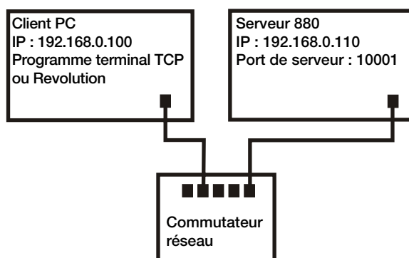
Illustration 9-2. Connexion entre un ordinateur et un serveur Ethernet d'indicateur 880 via un routeur ou un commutateur réseau
