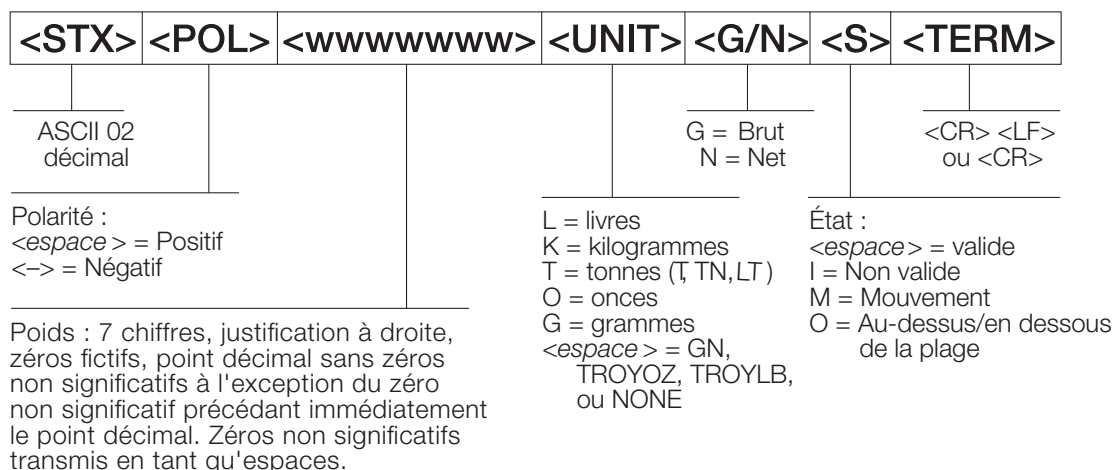
Illustration 10-1. Format de flux de données série – RS-232 et RS-422
