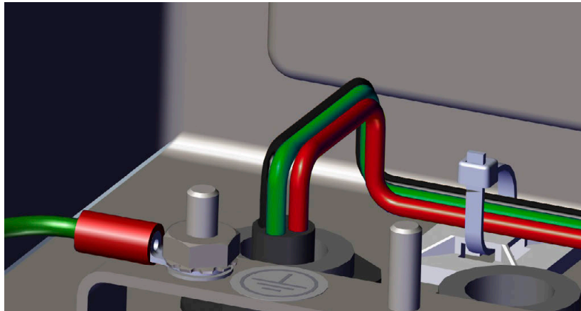
Illustration 2-21. Acheminement du cordon d'alimentation CC
