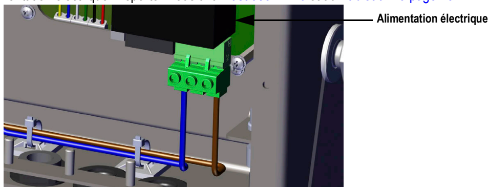
Illustration 2-20. Branchement du câble d'alimentation en courant alternatif
