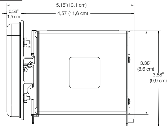
Illustration 2-1. Dimensions de l'indicateur 880 à boîtier pour installation à panneau
