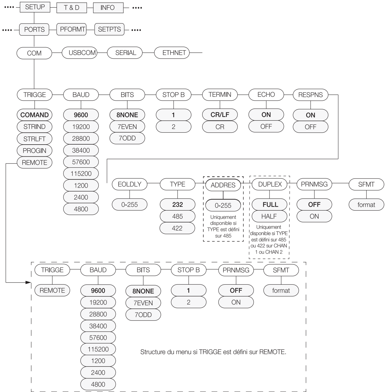
Illustration 3-12. Structures des menus Com, USBCOM, Canal carte série 1 et 2
