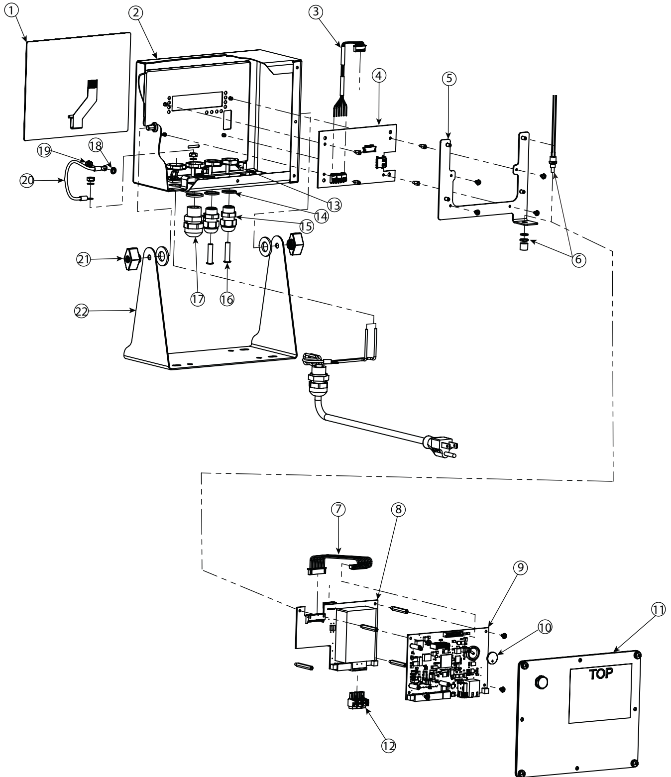
Illustration 2-32. Schéma - pièces de rechange pour indicateur 880 à boîtier universel
