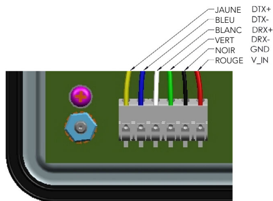
Illustration 2-8. Détail des fils du faisceau de câbles
