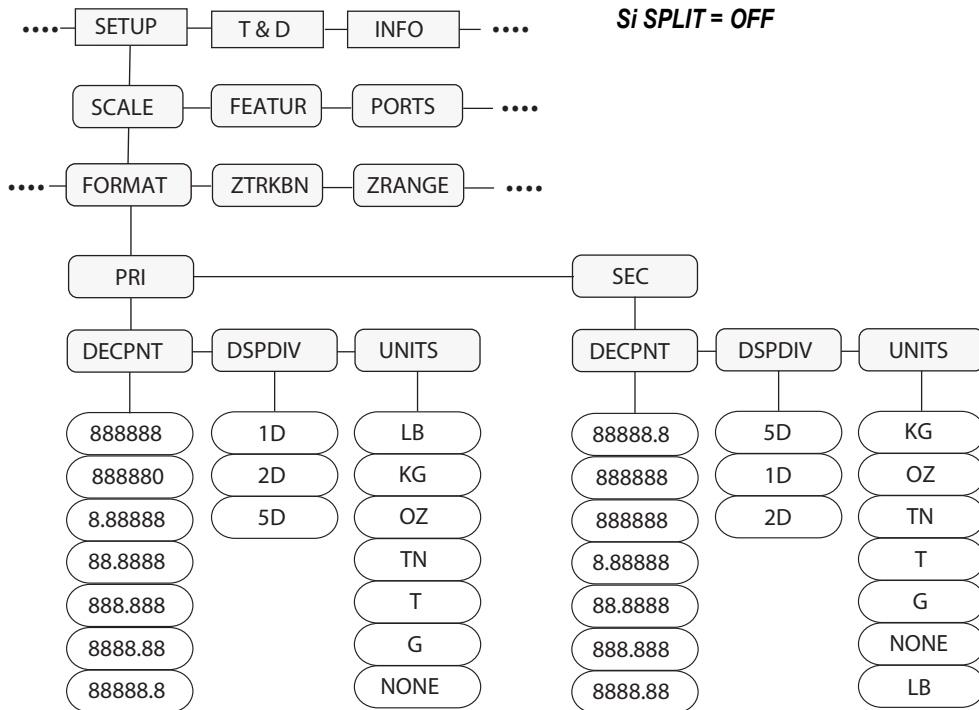
Illustration 3-6. Structure du menu Format avec Split défini sur Off
