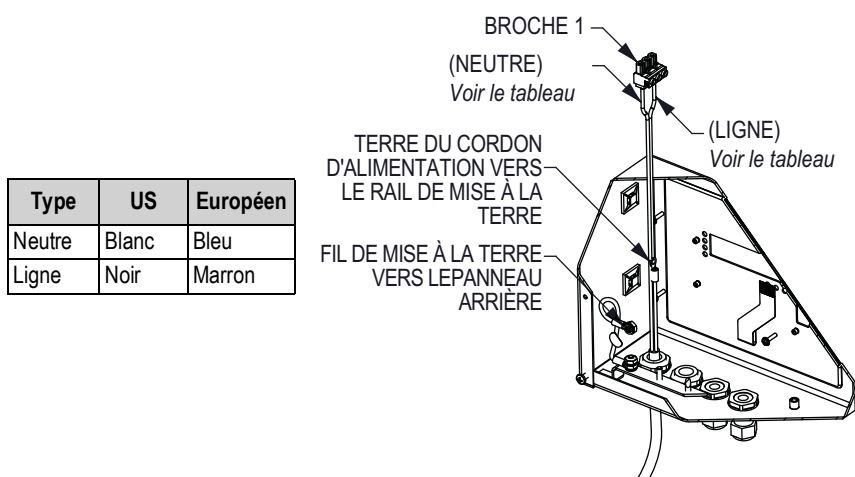
Illustration 2-19. Mise à la terre
