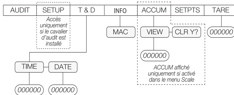
Illustration 3-2. Structure du menu de l'indicateur 880
