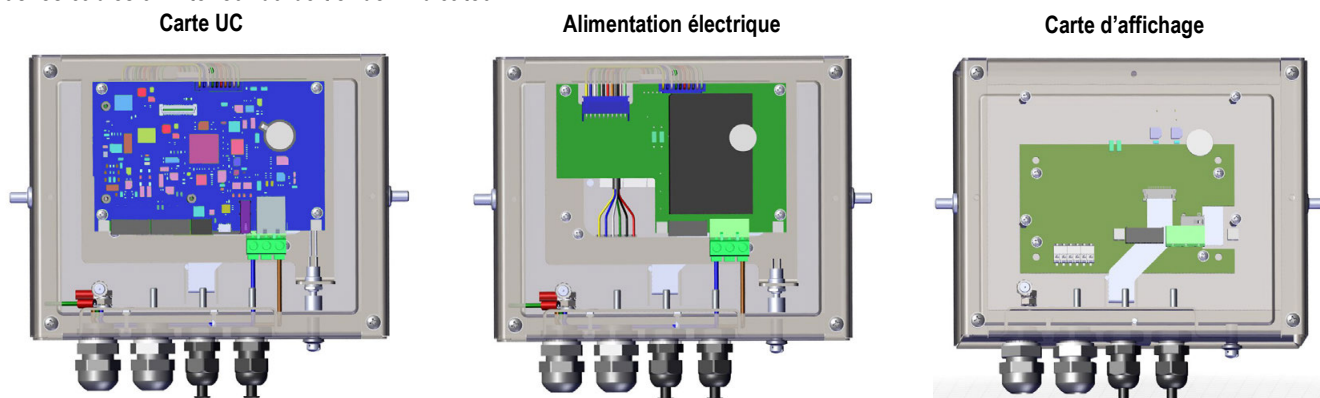
Illustration 2-16. Remplacement de cartes dans un boîtier universel d'indicateur 880
