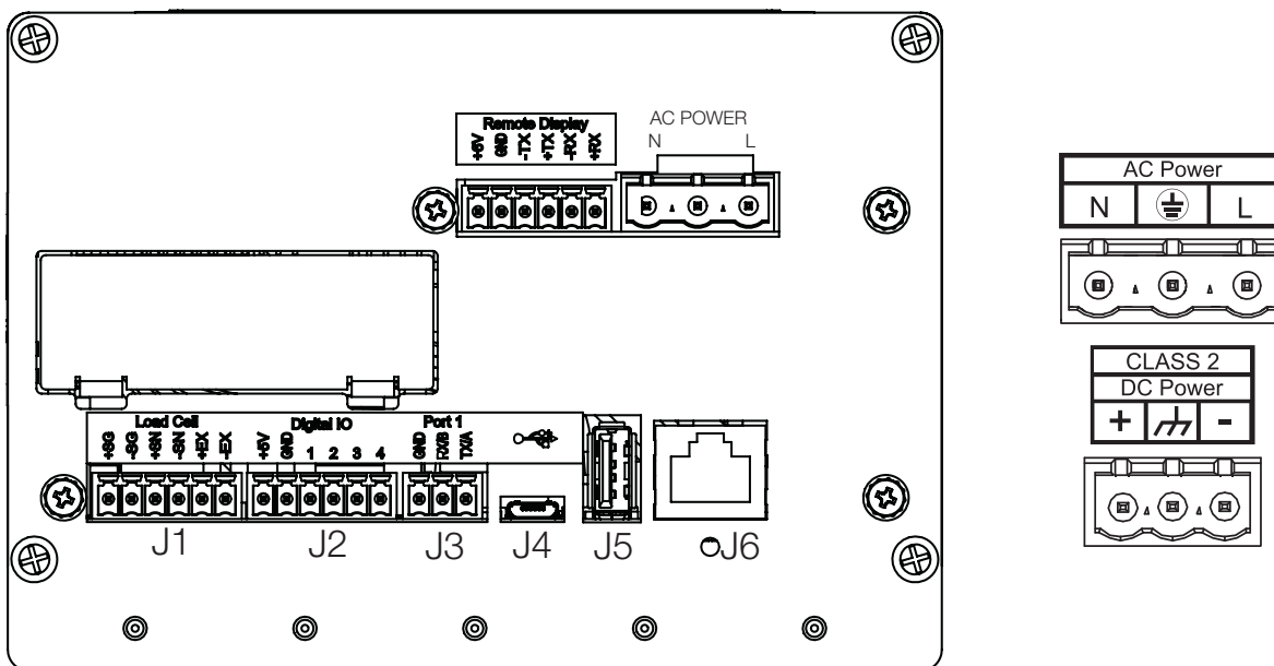
Illustration 2-17. Emplacement du raccordement électrique
