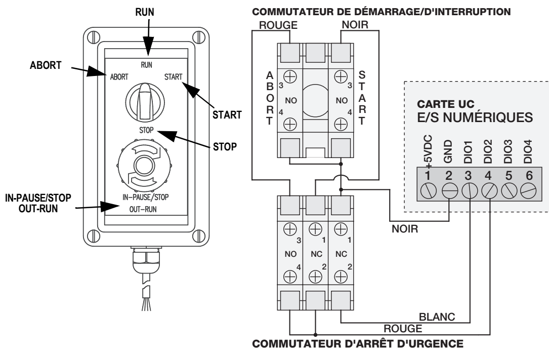
Illustration 8-1. Exemple de schéma de câblage et de commutateur de mise en lots
