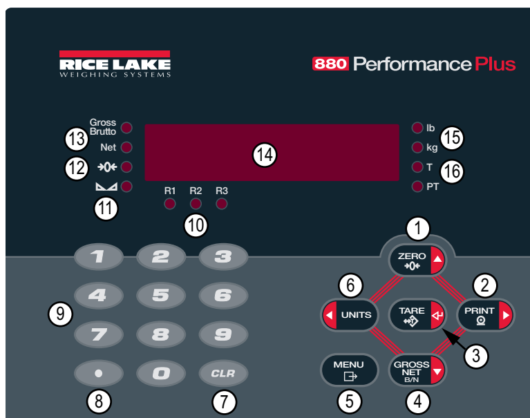
Illustration 1-1. Module d'affichage du panneau frontal de l'indicateur 880 (modèle universel illustré)
