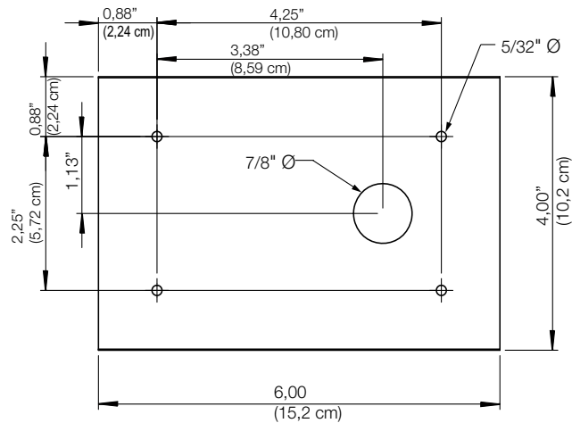
Illustration 2-2. Schéma de perçage des trous
