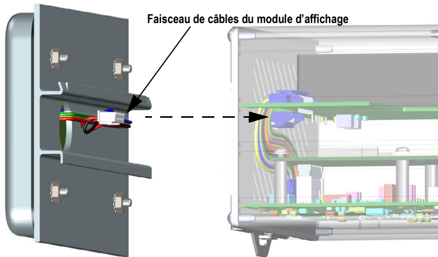
Illustration 2-7. Faisceau de câbles du module d'affichage
