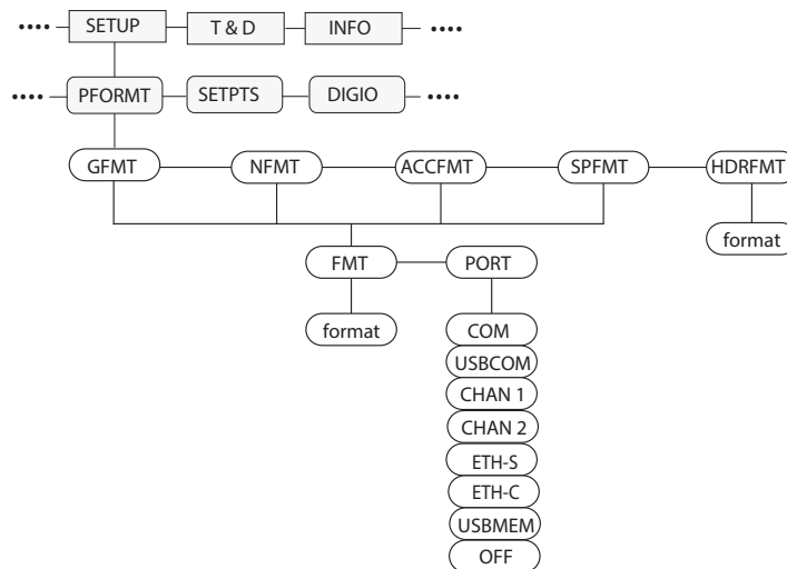
Illustration 3-16. Structure du menu de format d'impression
