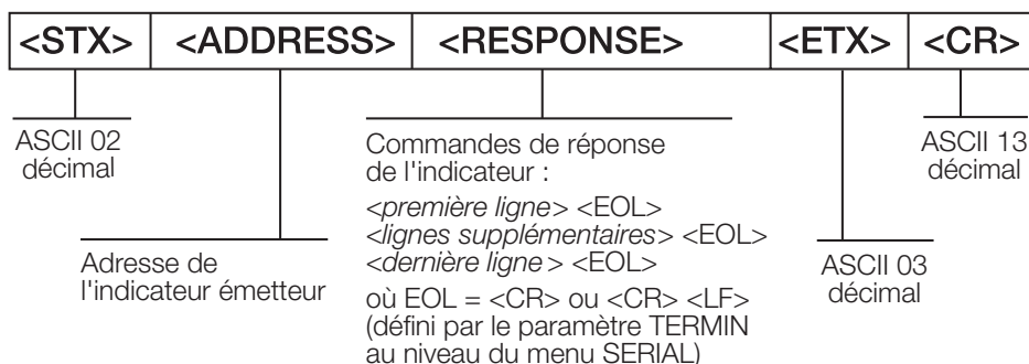
Illustration 10-3. Format de données pour les réponses RS-485
