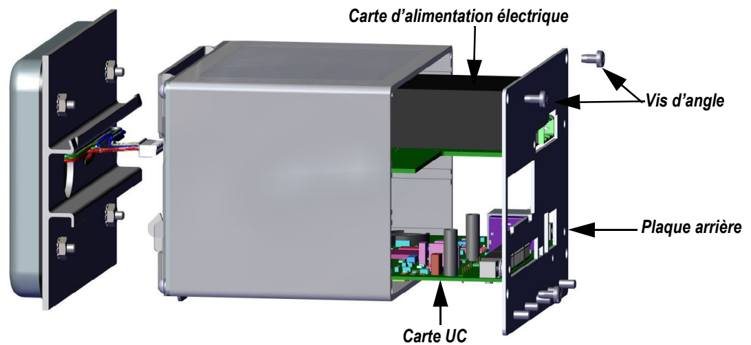
Illustration 2-11. Cartes extraites du boîtier
