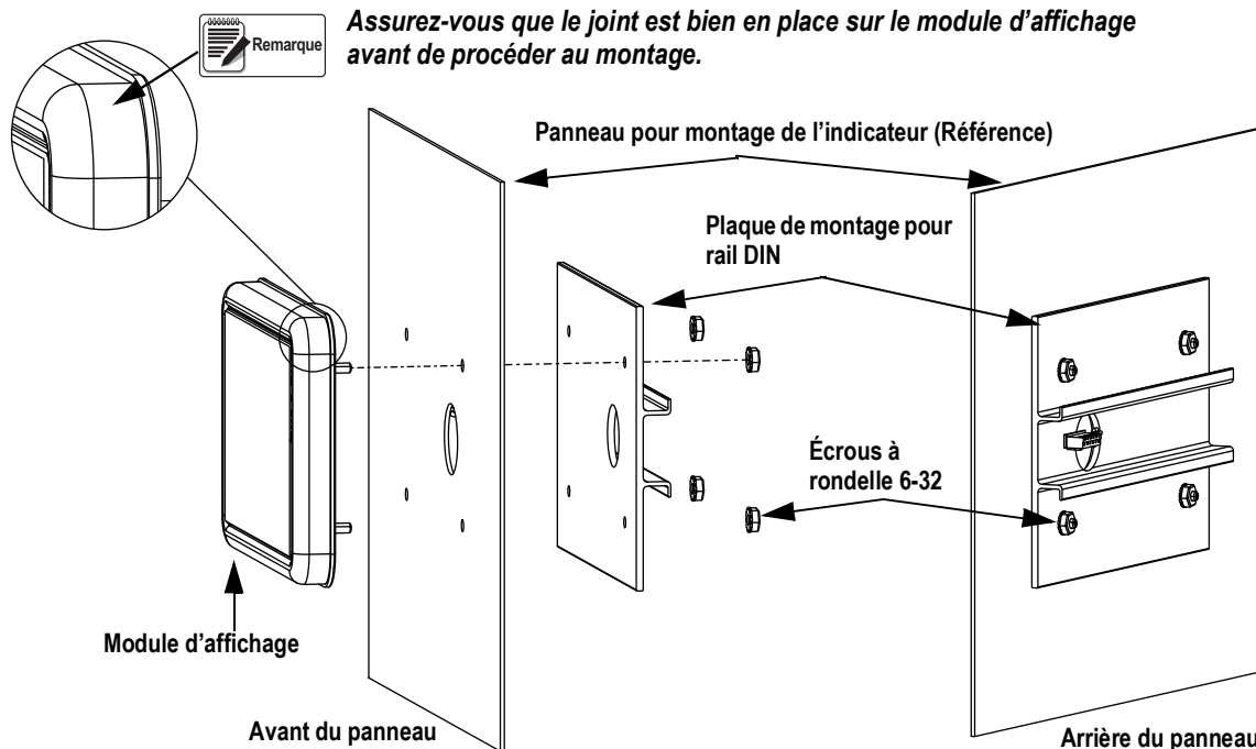
Illustration 2-3. Montage du module d'affichage
