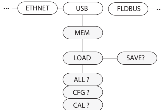
Illustration 3-14. Structure de menu USB Host (menu d'hôte USB)
