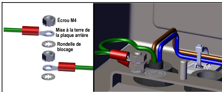
Illustration 2-18. Empilage de mise à la terre pour alimentation CA
