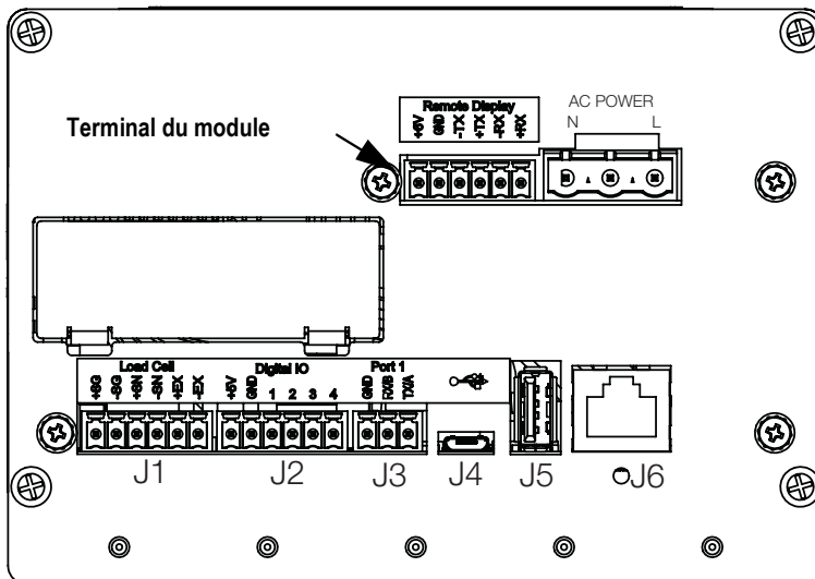
Illustration 2-5. Installation du contrôleur à distance
