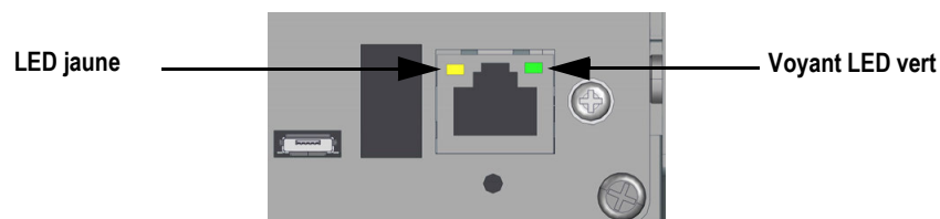
Illustration 2-23. Connecteur Ethernet RJ45 – Installation à panneau
