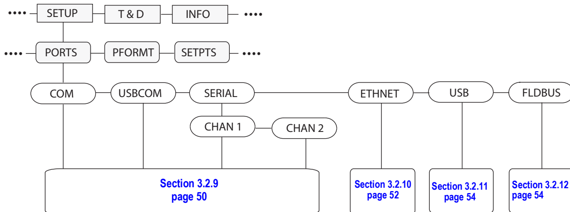
Illustration 3-11. Structure du menu Ports
