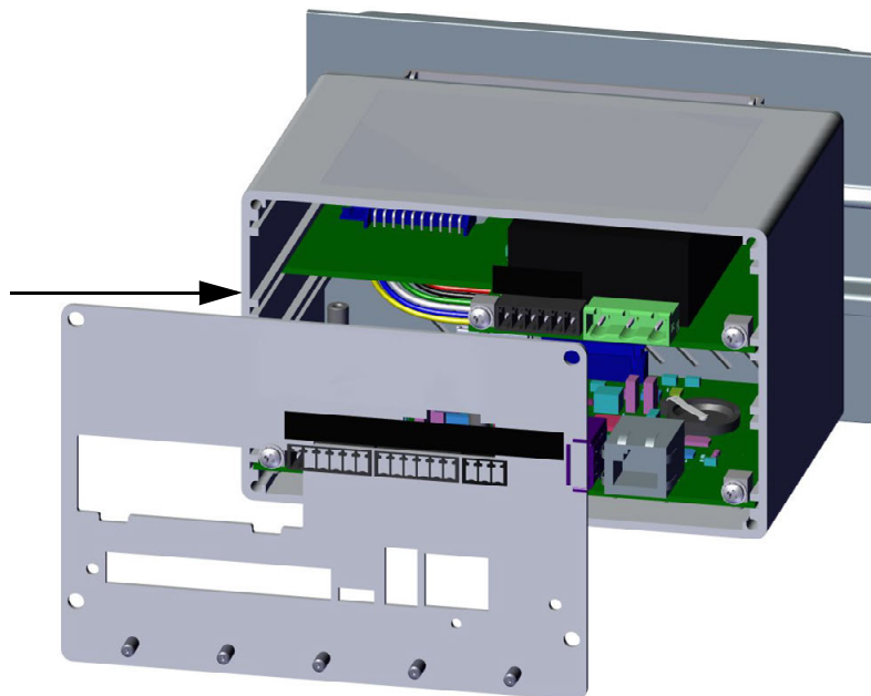
Illustration 2-12. Cartes installées dans le boîtier du contrôleur
