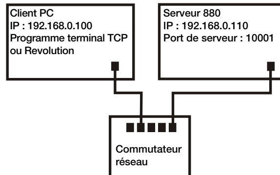
Illustration 9-3. Connexion à un hôte distant
