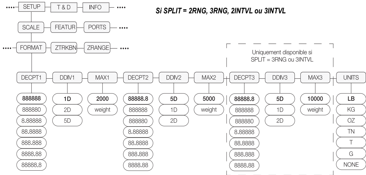
Illustration 3-7. Structure du menu Format avec Split 2RNG, 3RNG 2INTVL ou 3INTVL
