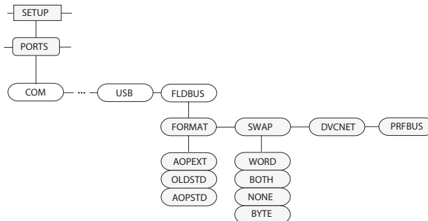
Illustration 3-15. Paramètres de menu de bus de terrain
