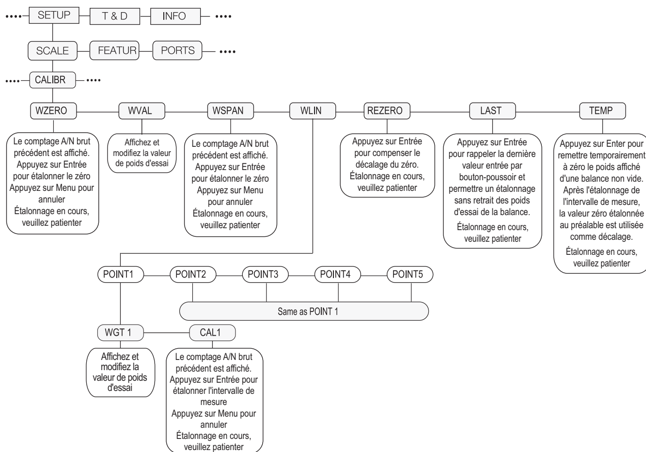
Illustration 4-1. Menu d'étalonnage (CALIBR)
