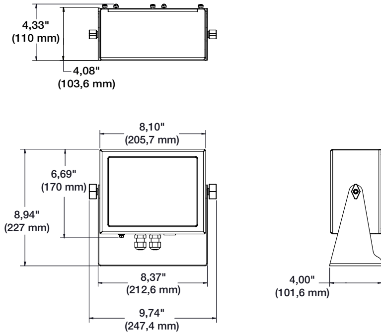
Illustration 2-13. Dimensions du boîtier universel
