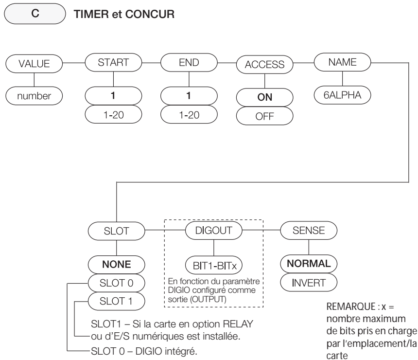
Illustration 3-20. Structure du menu de points de consigne – Structure C
