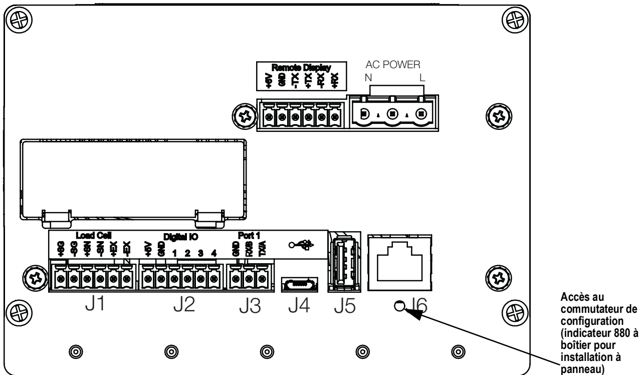
Illustration 3-1. Vue arrière – Accès au commutateur de configuration
