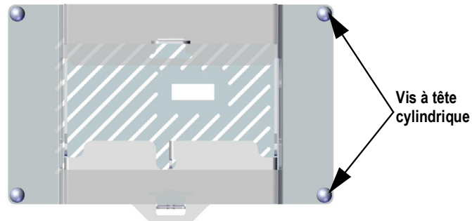
Illustration 2-28. Emplacement des vis du support de rail DIN
