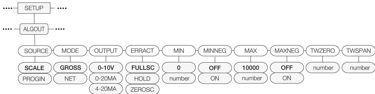
Illustration 3-23. Menu de sortie analogique
