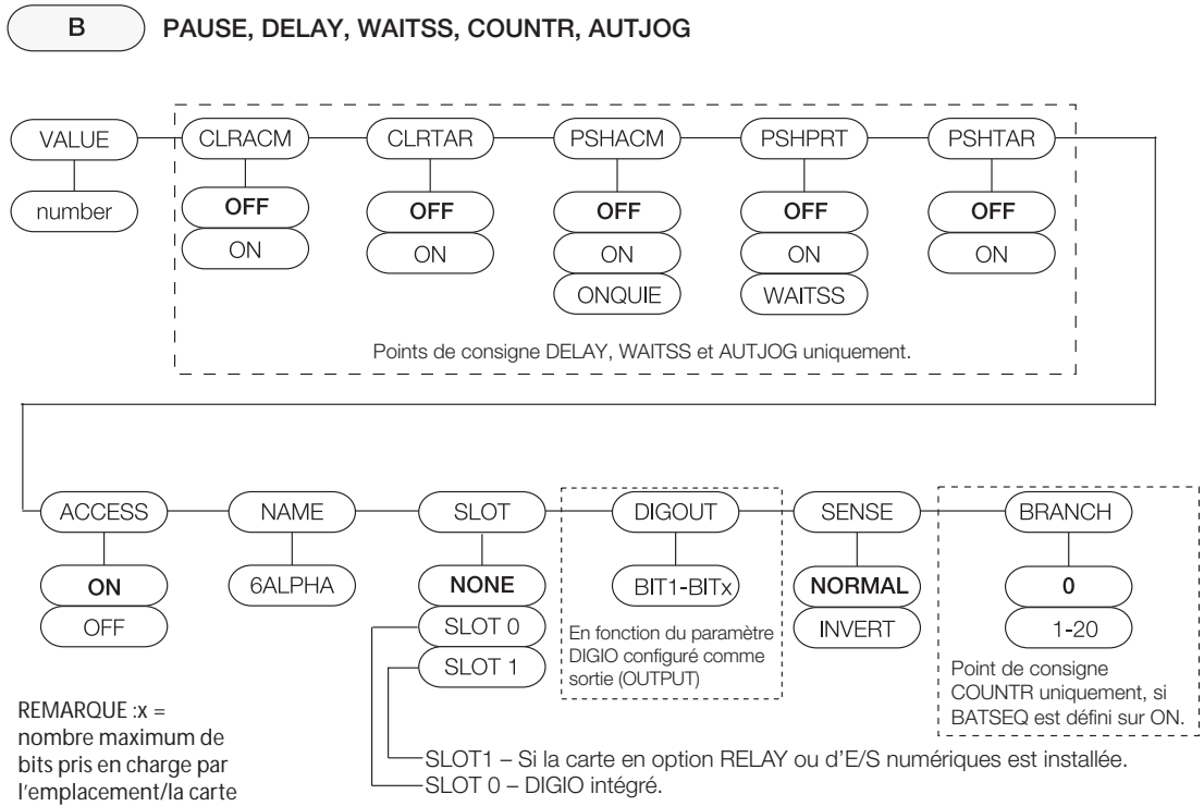
Illustration 3-19. Structure du menu de points de consigne – Structure B
