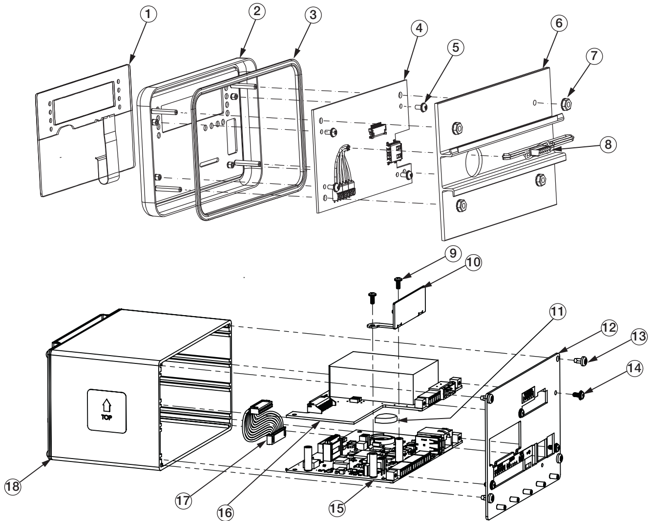
Illustration 2-31. Illustration des pièces de l'indicateur 880
