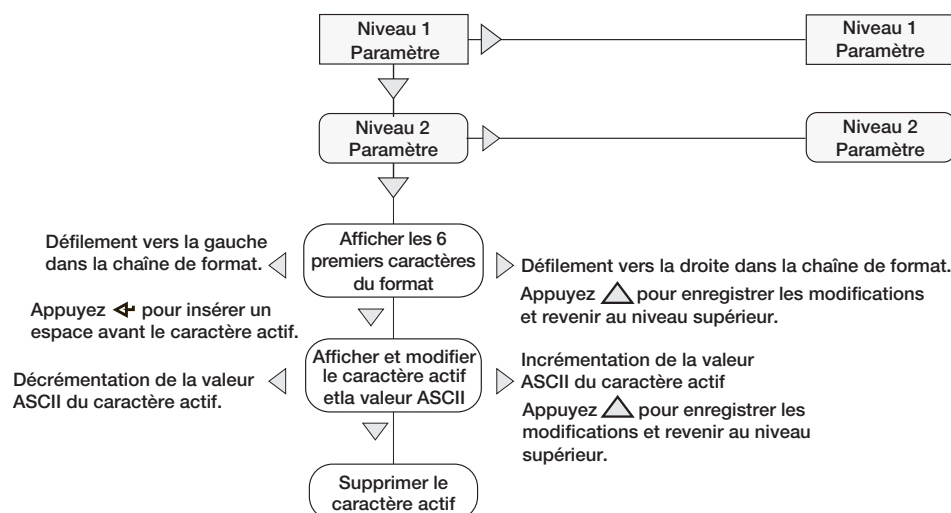
Illustration 1-3. Procédure de modification de valeur numérique
