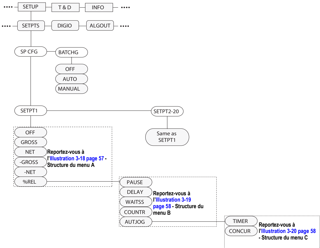
Illustration 3-17. Structure du menu de points de consigne
