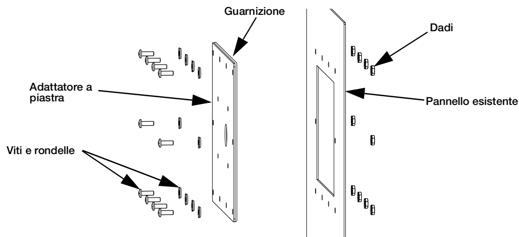
Figura 4. Installazione dell'adattatore a piastra
