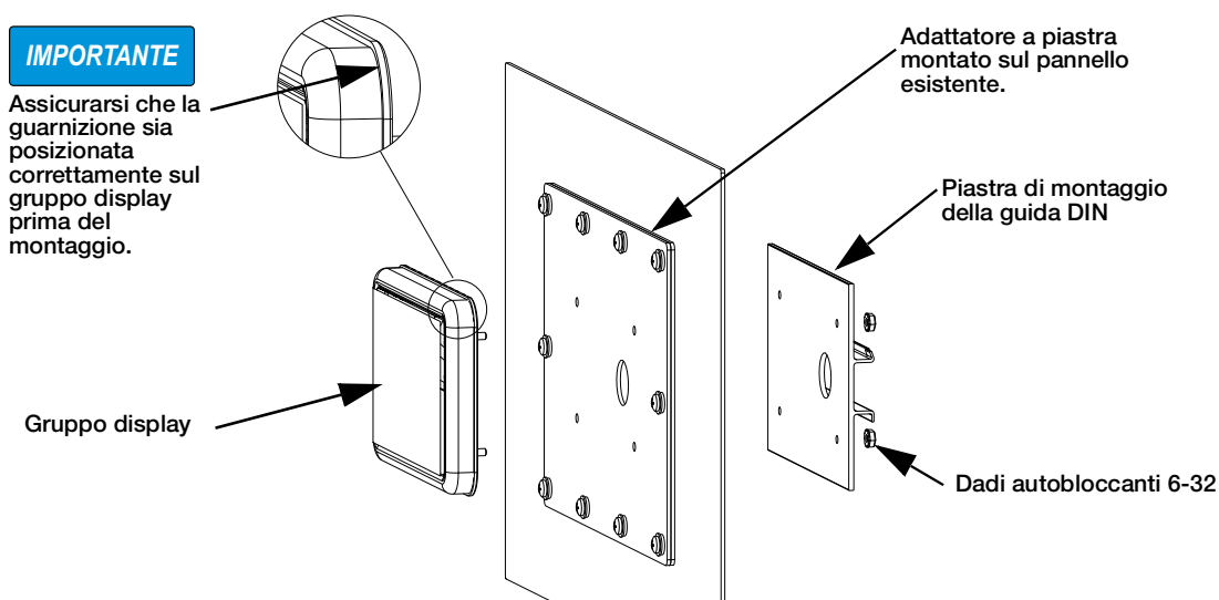
Figura 5. Installazione del display
