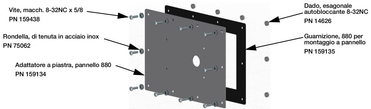
Figura 1. Parti per l'opzione di retrofit del pannello
