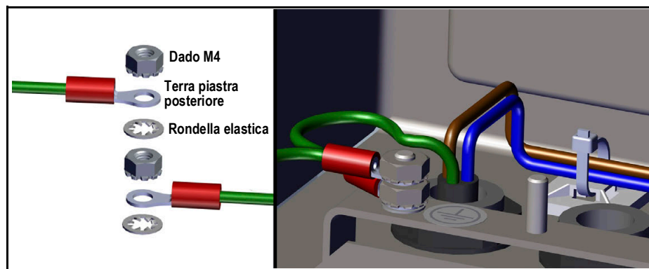
Figura 2-18. Componenti per la messa a terra AC
