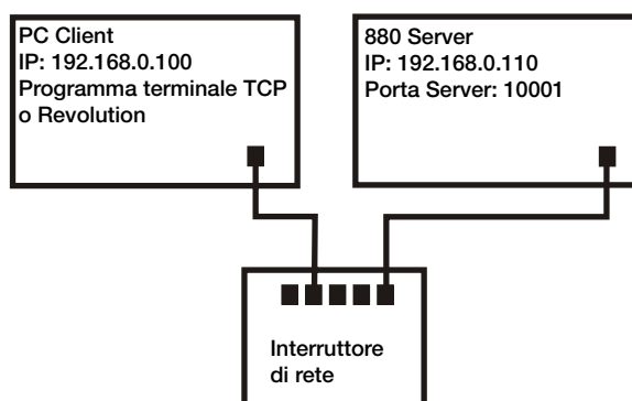
Figura 9-2. Connessione dal computer a Ethernet dell'880 attraverso uno switch di rete o un router
