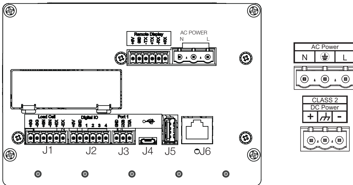
Figura 2-17. Posizione dei collegamenti dell'alimentazione
