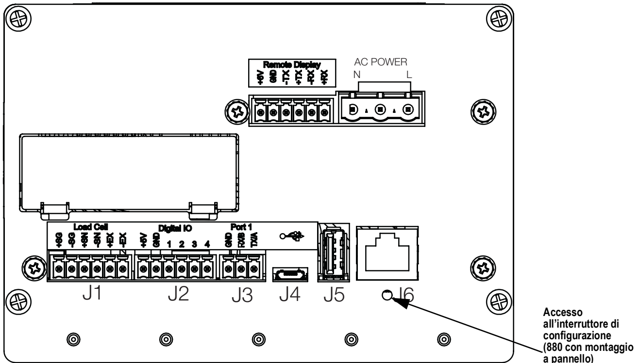
Figura 3-1. Vista posteriore – Accesso all'interruttore di configurazione
