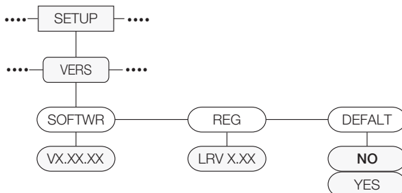
Figura 3-21. Struttura del menu Version
