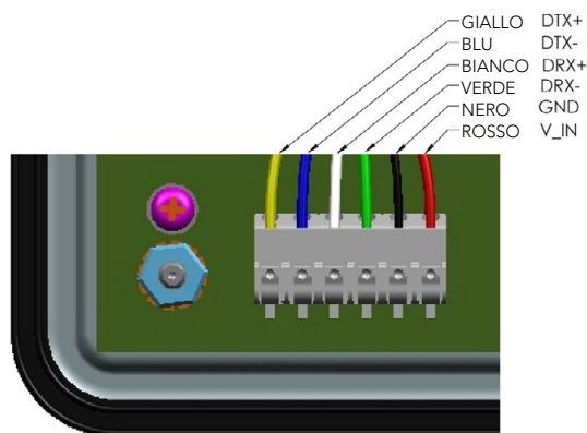
Figura 2-8. Dettaglio del collegamento del fascio di cavi
