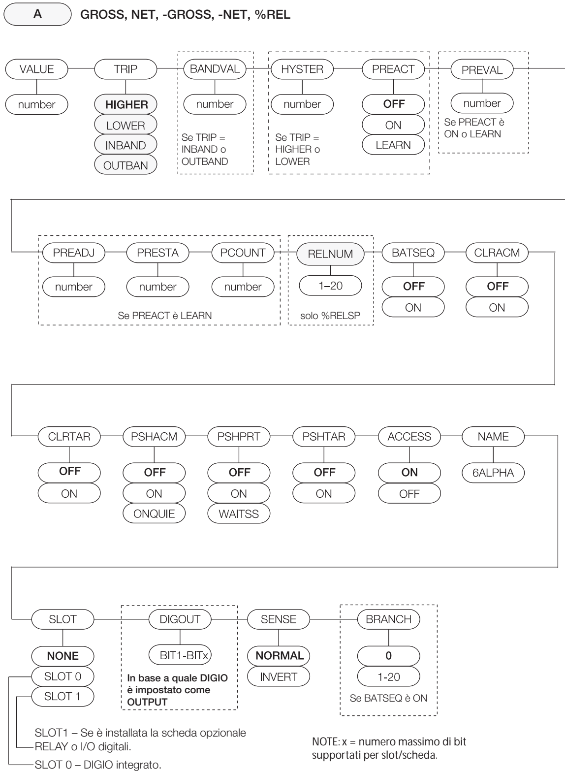
Figura 3-18. Struttura del menu Setpoint – Layout A
