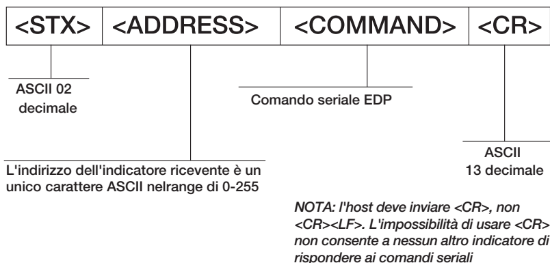
Figura 10-2. Formati dei dati di trasmissione RS-485
