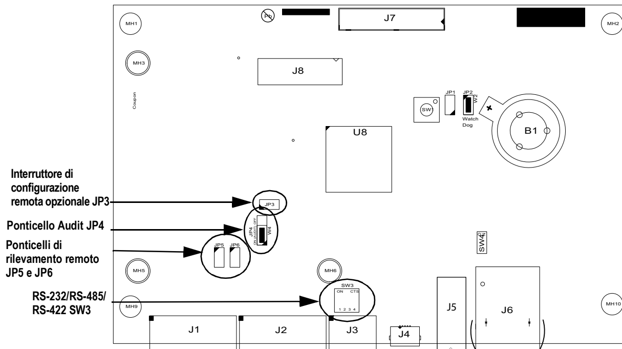
Figura 2-24. Scheda CPU dell'880
