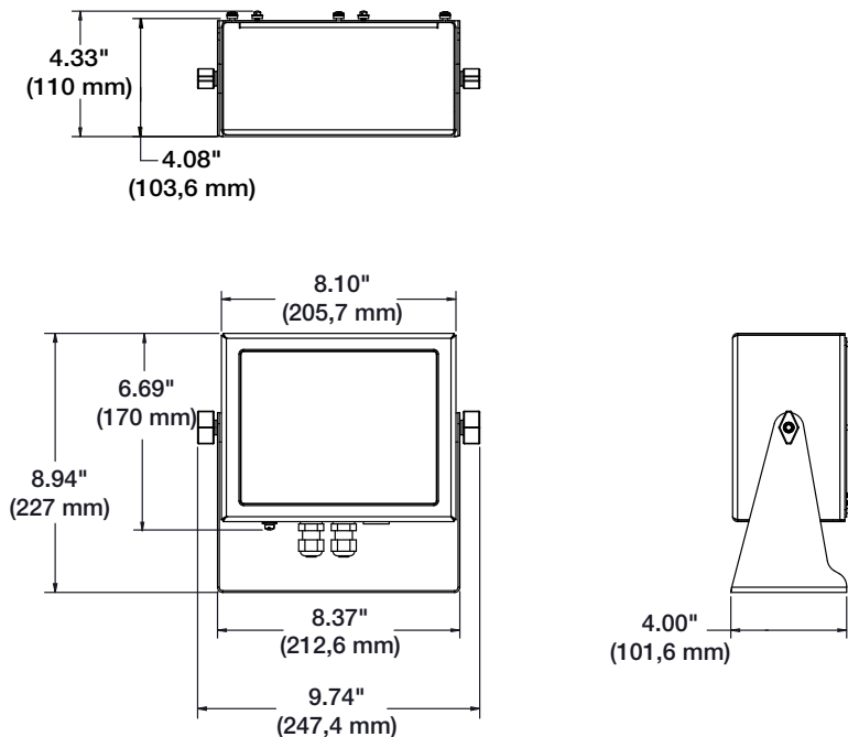
Figura 2-13. Dimensioni del supporto universale
