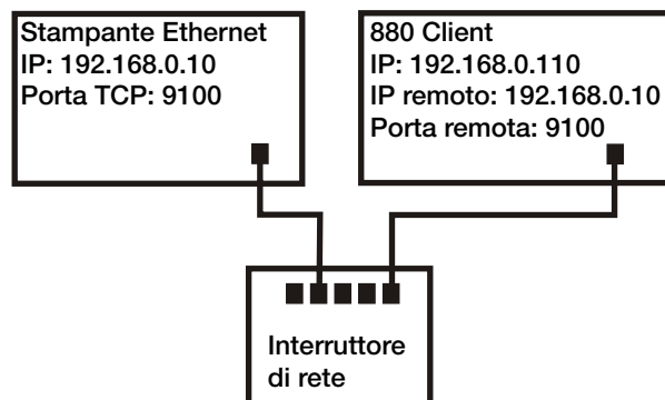
Figura 9-3. Connessione a un host remoto
