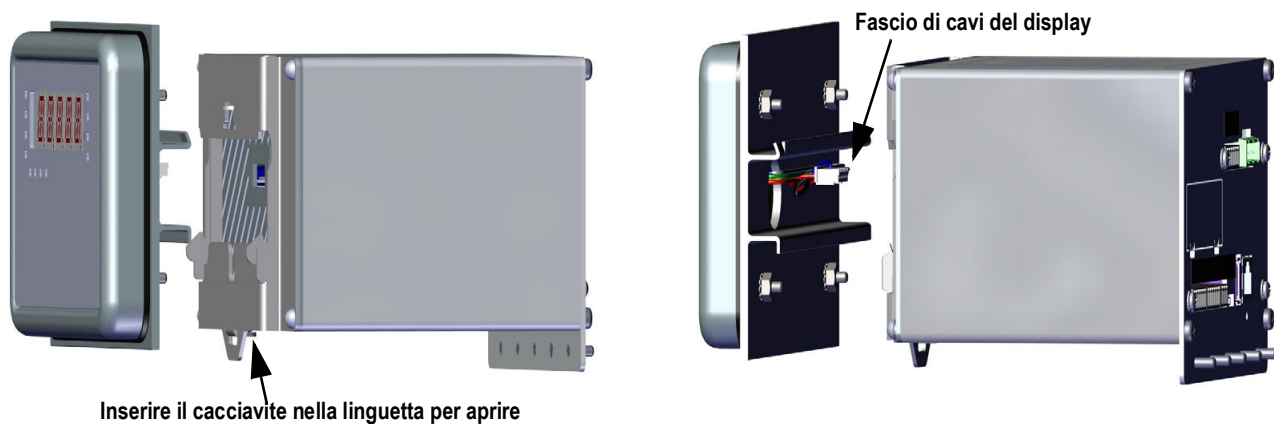
Figura 2-4. Installazione del gruppo controller
