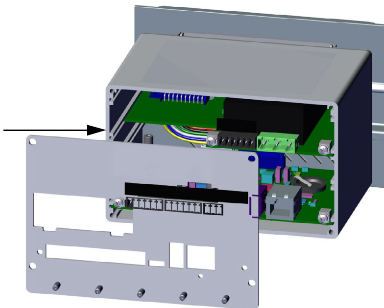
Figura 2-12. Schede installate nell'involucro del gruppo controller
