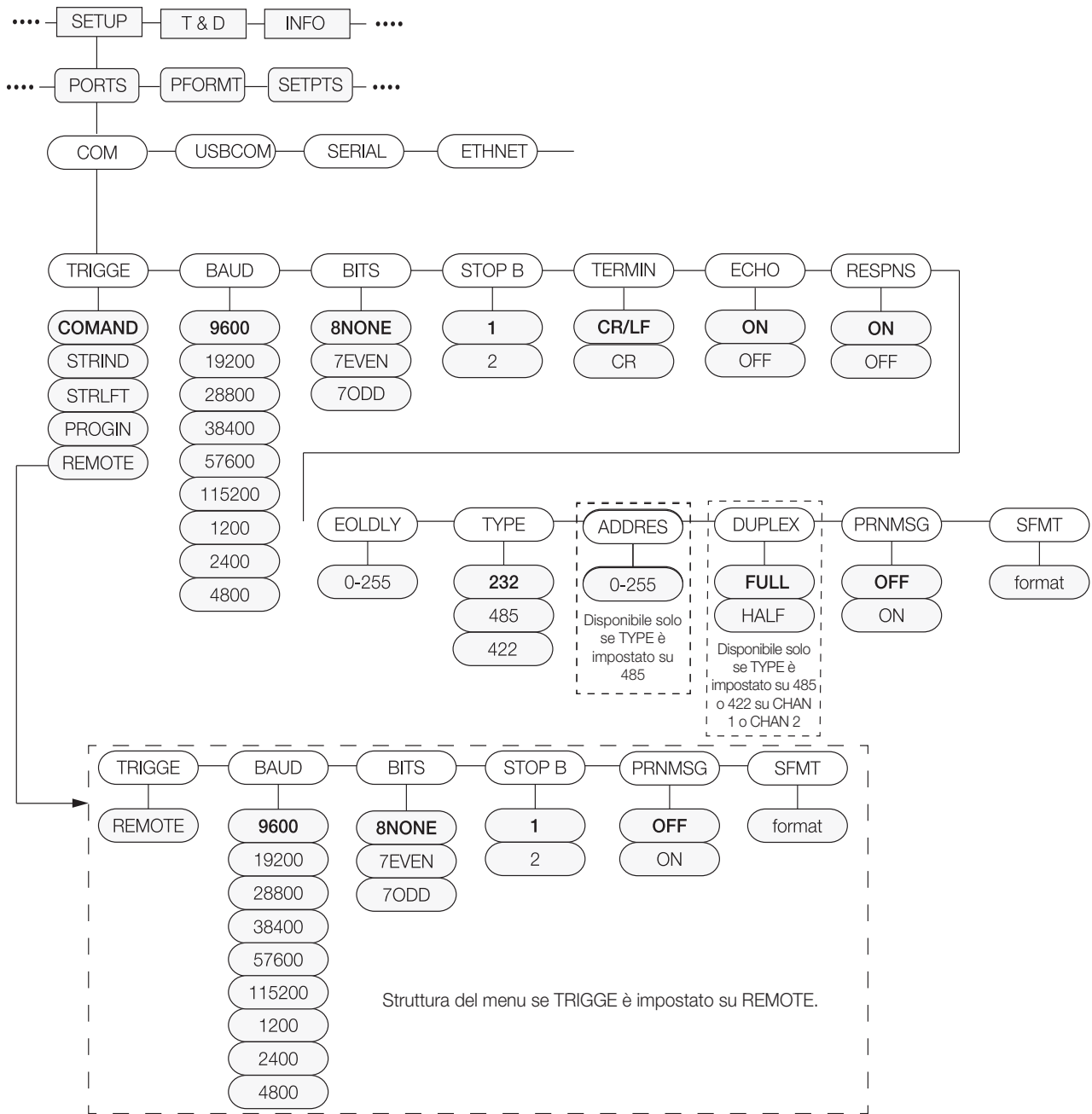
Figura 3-12. Strutture dei menu Com, USBCOM, Canale 1 e 2 scheda seriale
