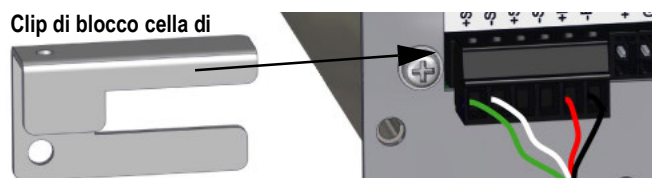
Figura 2-26. Fissaggio della clip di blocco della cella di carico
