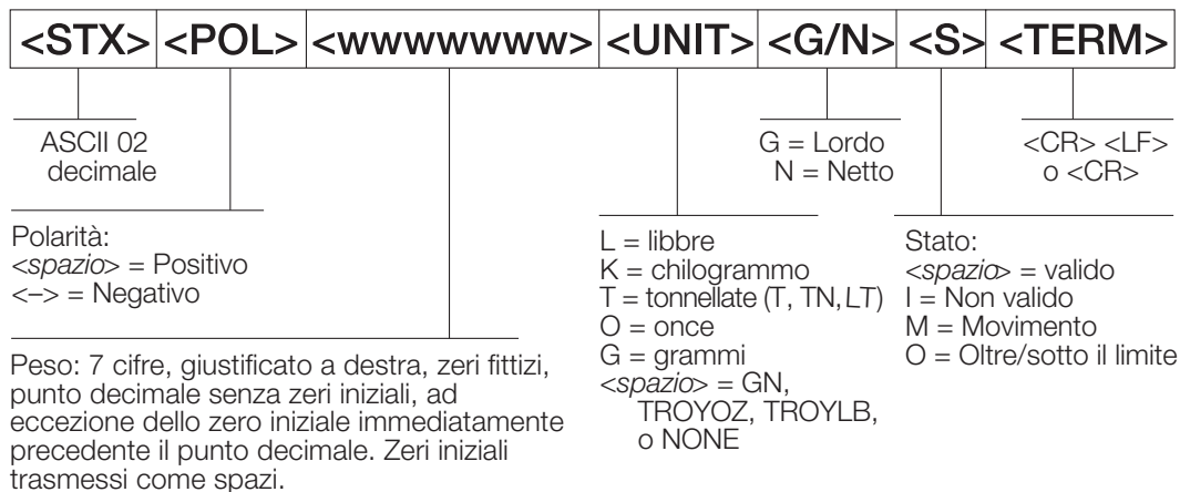
Figura 10-1. Formato dati di flusso seriali – RS-232 e RS-422
