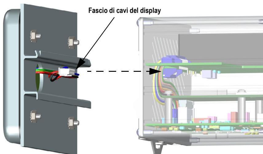
Figura 2-7. Collegamento del fascio di cavi del display
