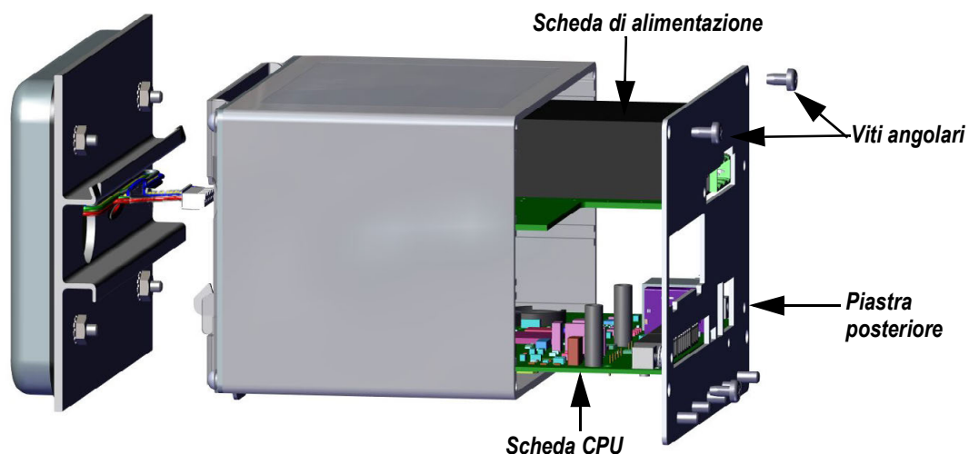
Figura 2-11. Schede rimosse dall'involucro
