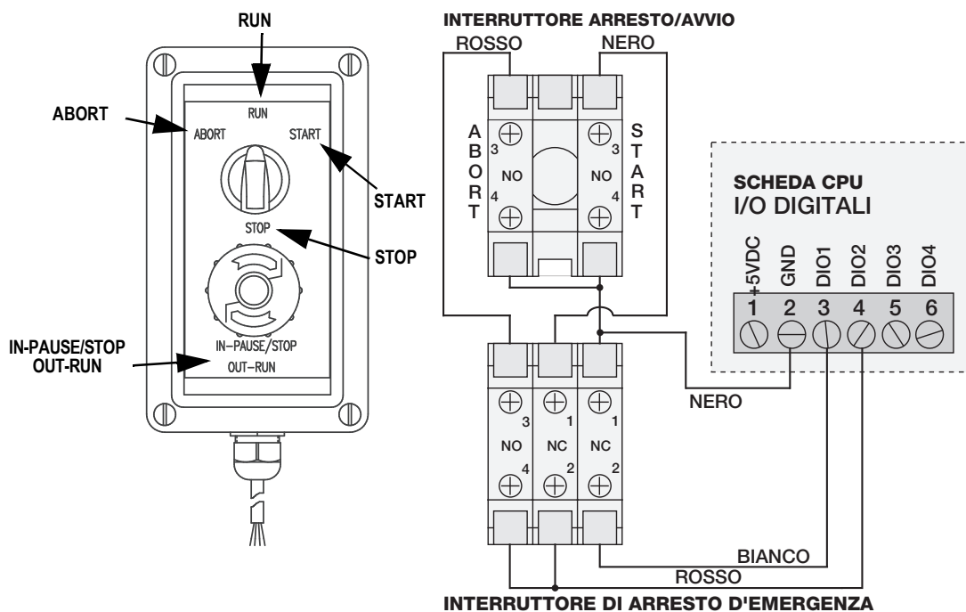
Figura 8-1. Esempio di interruttore di batch e schema di cablaggio
