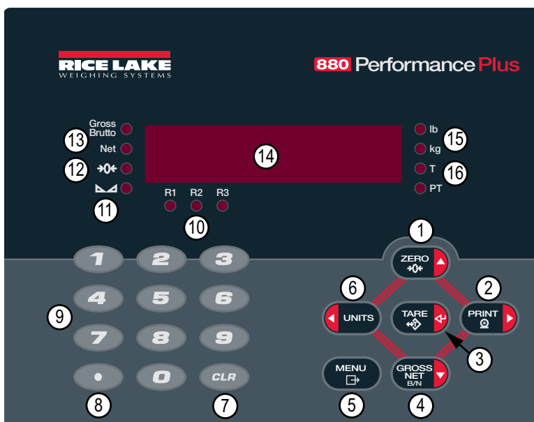
Figura 1-1. Display del pannello frontale 880 (è raffigurato il modello universale)
