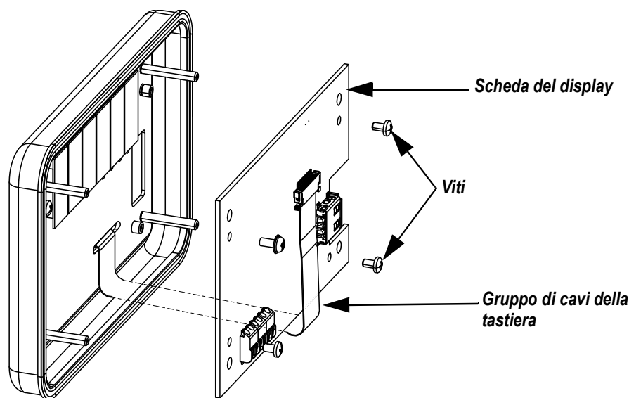
Figura 2-10. Scheda del display
