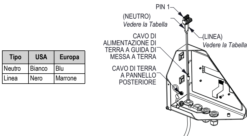
Figura 2-19. Collegamenti di messa a terra
