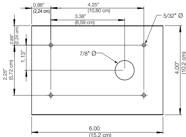
Figura 2-2. Schema per l'esecuzione dei fori
