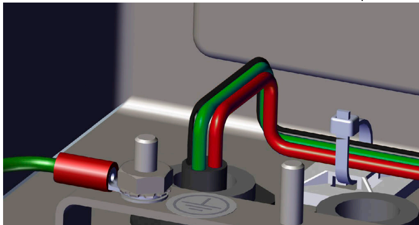
Figura 2-21. Posa del cavo di alimentazione DC
