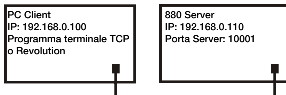
Figura 9-1. Connessione diretta da computer a Ethernet dell'880
