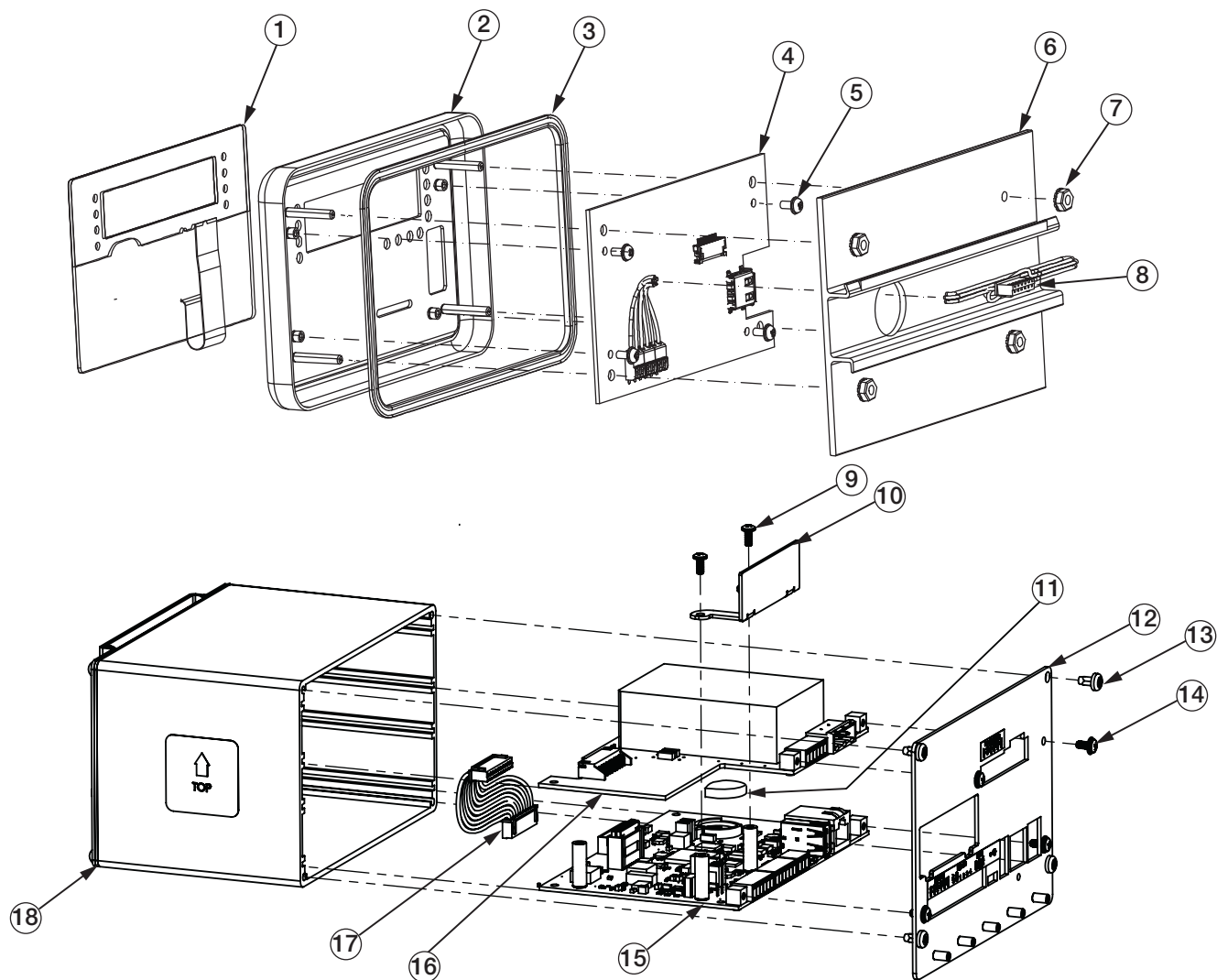
Figura 2-31. Illustrazione dei componenti dell'indicatore 880
