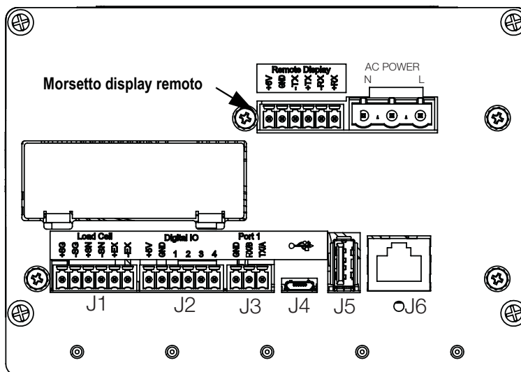
Figura 2-5. Montaggio del gruppo controller a distanza
