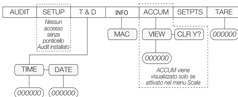
Figura 3-2. Struttura del menu dell'880
