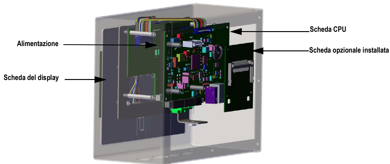
Figura 2-15. Posizioni delle schede nel supporto universale
