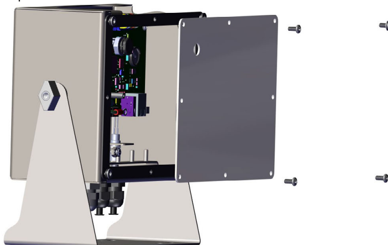
Figura 2-14. Rimozione della piastra posteriore del supporto universale
