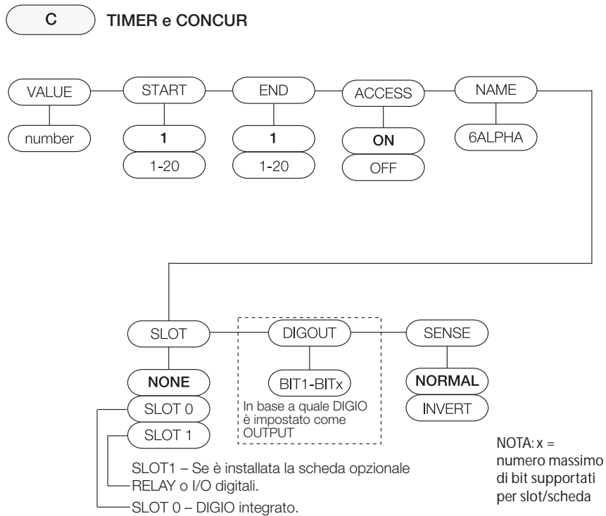
Figura 3-20. Struttura del menu Setpoint– Layout C
