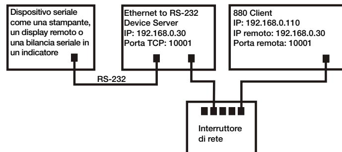
Figura 9-4. Streaming di dati su richiesta da Ethernet remoto a un server di dispositivi RS232
