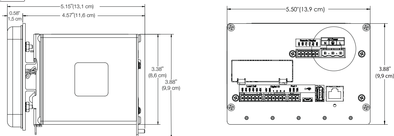
Figura 2-1. Dimensioni dell'indicatore 880 con montaggio a pannello
