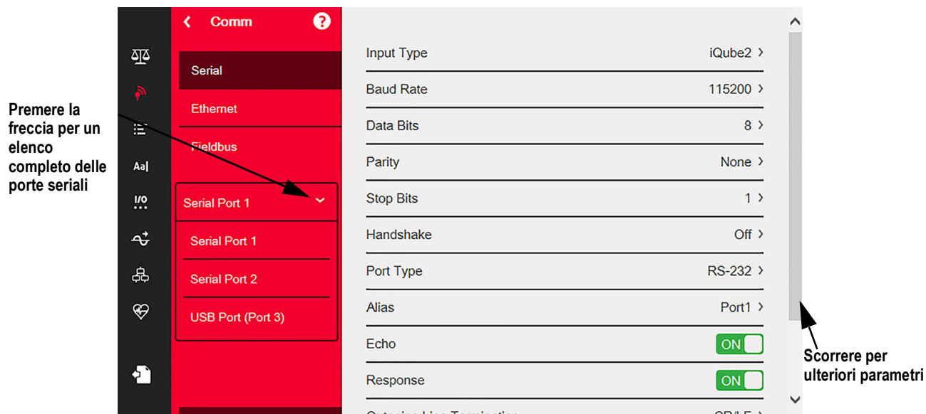
Figura 5-2. Schermata del menu Serial
