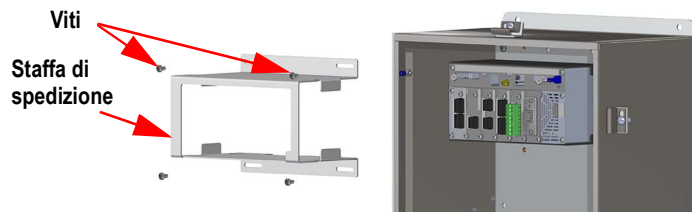
Figura 2-9. Rimuovere la staffa di spedizione
