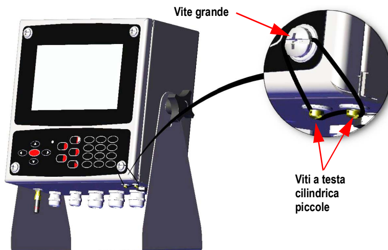
Figura 2-7. Sigillare la porta anteriore (supporto universale)
