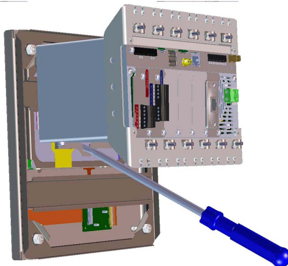
Figura 2-21. Rimozione del gruppo controller
