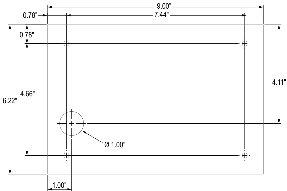
Figura 2-16. Dimensioni della versione da 7" con montaggio a pannello solo touch
