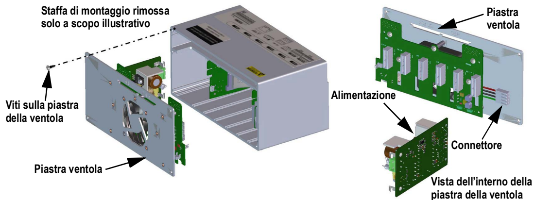
Figura 2-37. Rimozione dell'alimentatore
