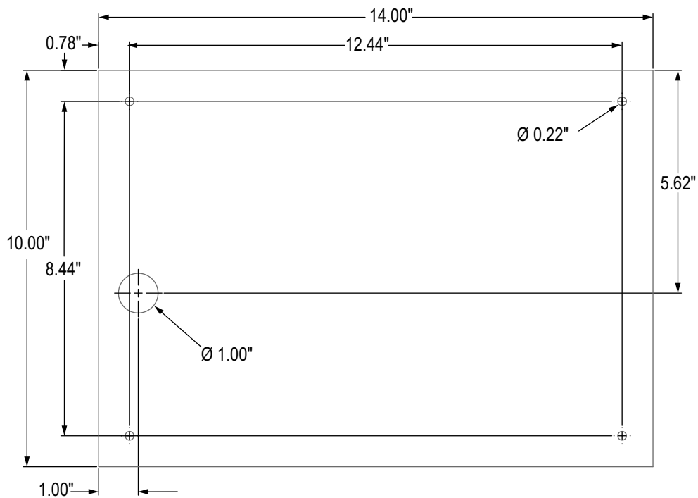
Figura 2-17. Dimensioni della versione da 12" con montaggio a pannello solo touch
