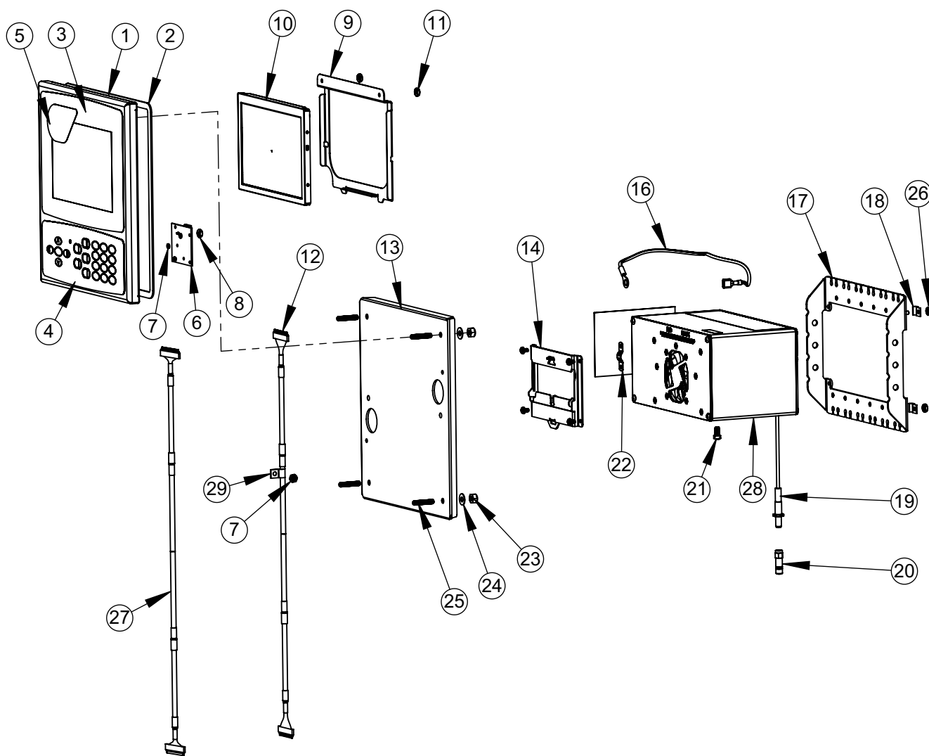
Figura 2-43. Componenti per la riparazione dell'indicatore da 7" con montaggio a pannello
