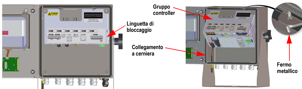
Figura 2-4. Rimozione del gruppo CPU – Involucro universale
