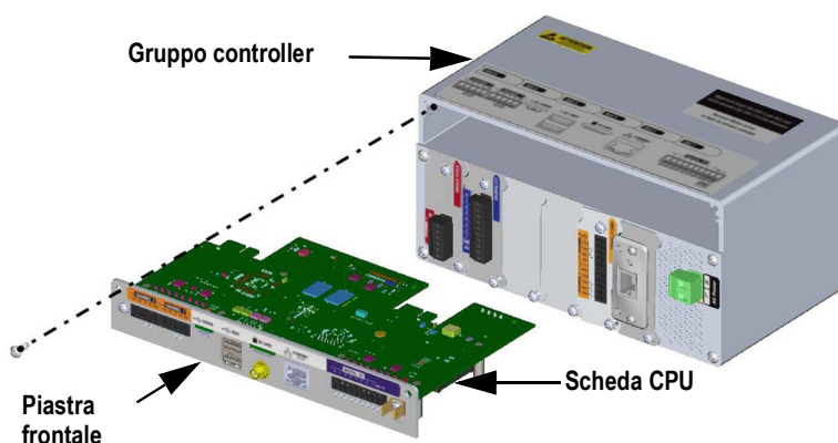
Figura 2-35. Rimozione della scheda CPU
