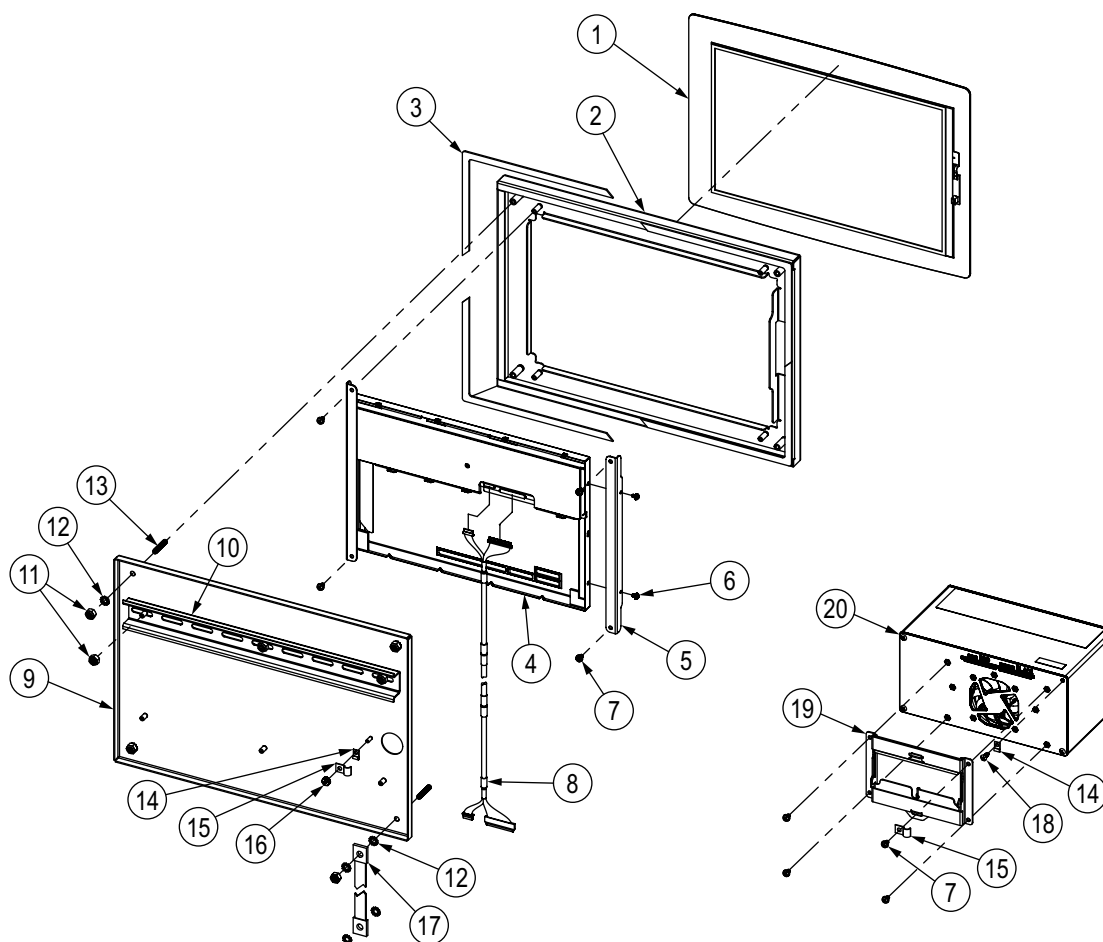
Figura 2-45. Componenti per la riparazione dell'indicatore da 12" con montaggio a pannello solo touch
