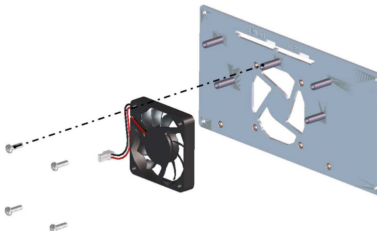
Figura 2-39. Rimozione della ventola
