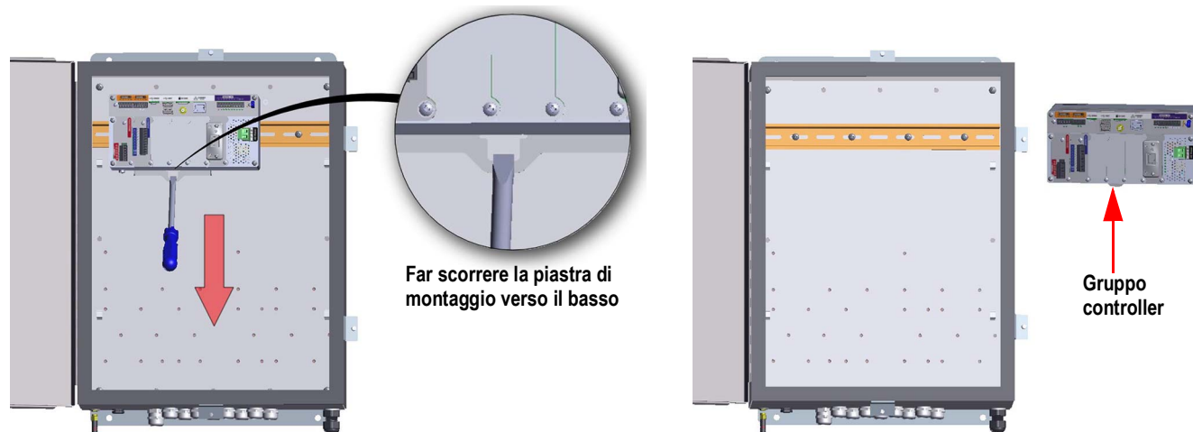
Figura 2-11. Rimuovere il gruppo controller - Montaggio a parete
