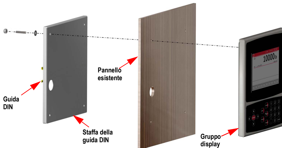
Figura 2-14. Installazione con montaggio a pannello
