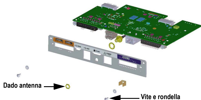
Figura 2-36. Scheda CPU e piastra frontale
