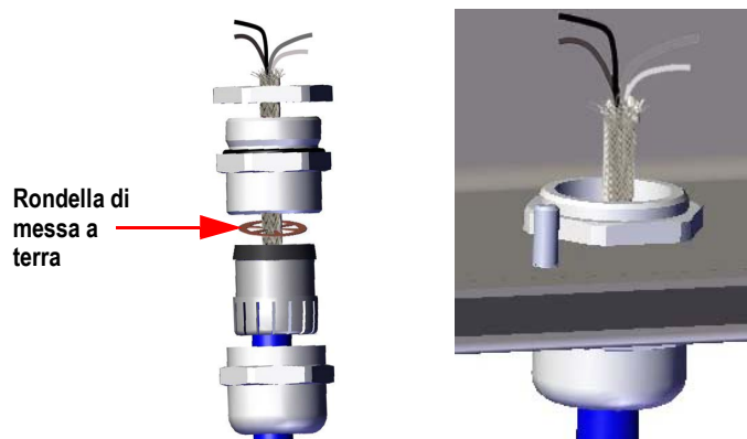
Figura 2-27. Messa a terra dell'involucro universale e a parete
