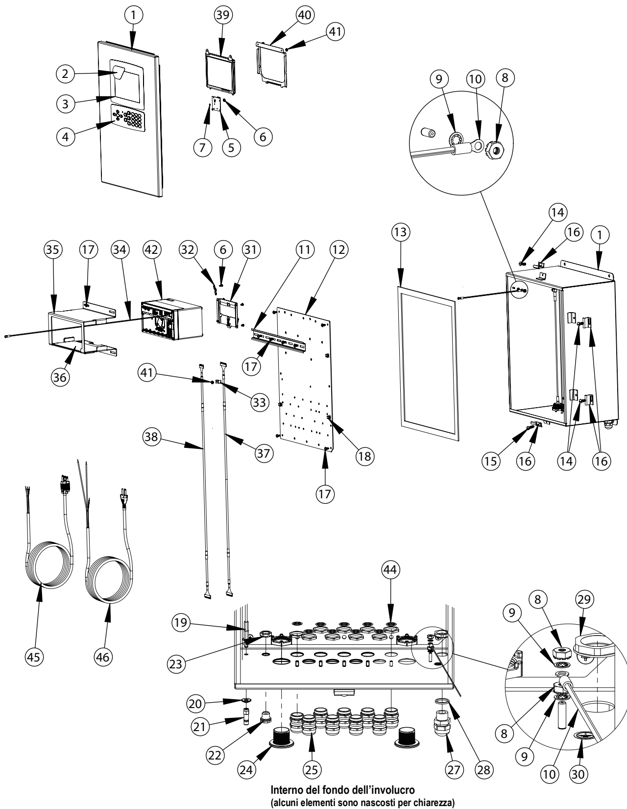
Figura 2-41. Componenti per la riparazione dell'indicatore con montaggio a parete
