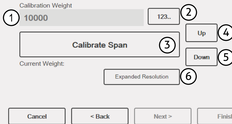
Figura 4-5. Calibrazione dello span
