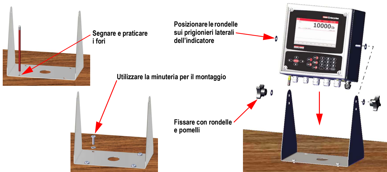
Figura 2-1. Montaggio involucro universale
