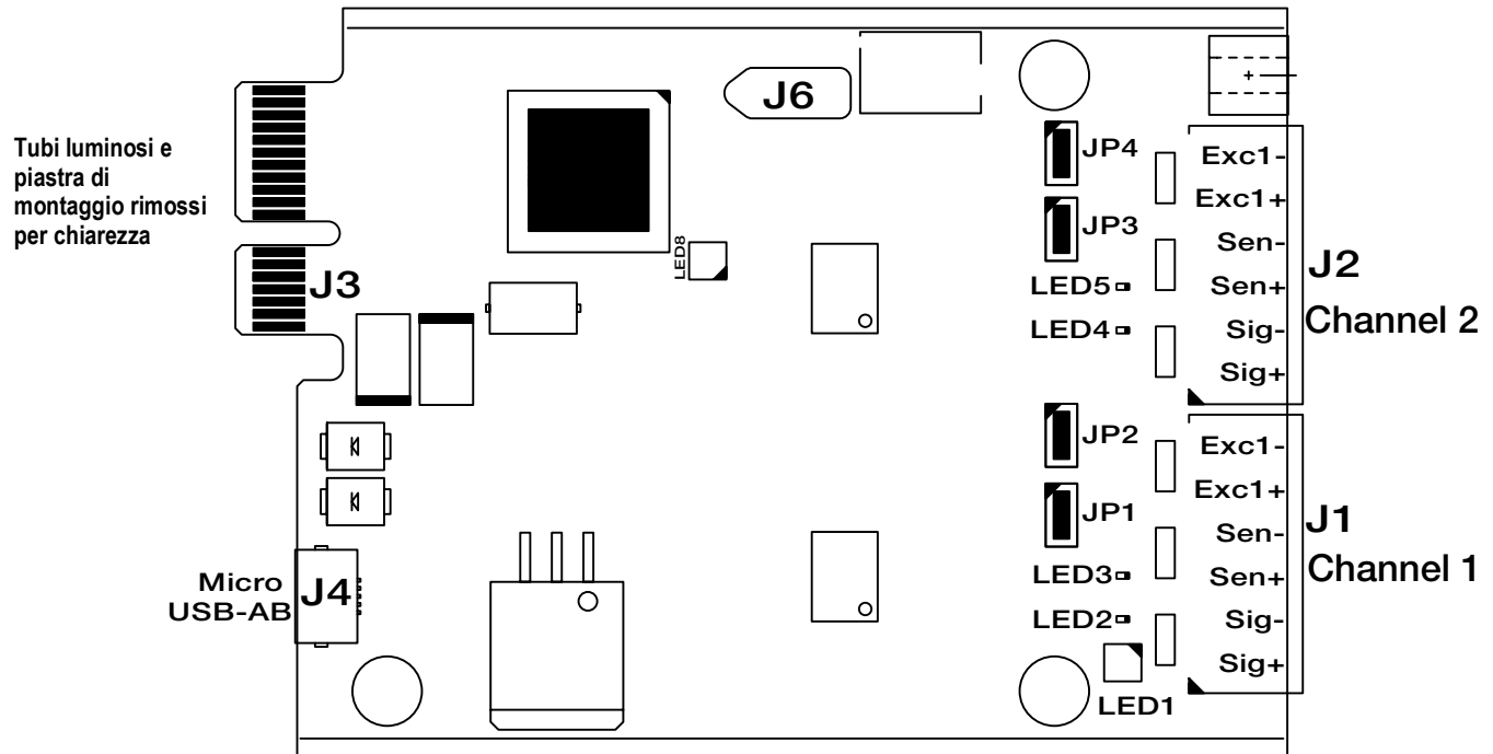
Figura 2-31. Schede della bilancia A/D singole e doppie
