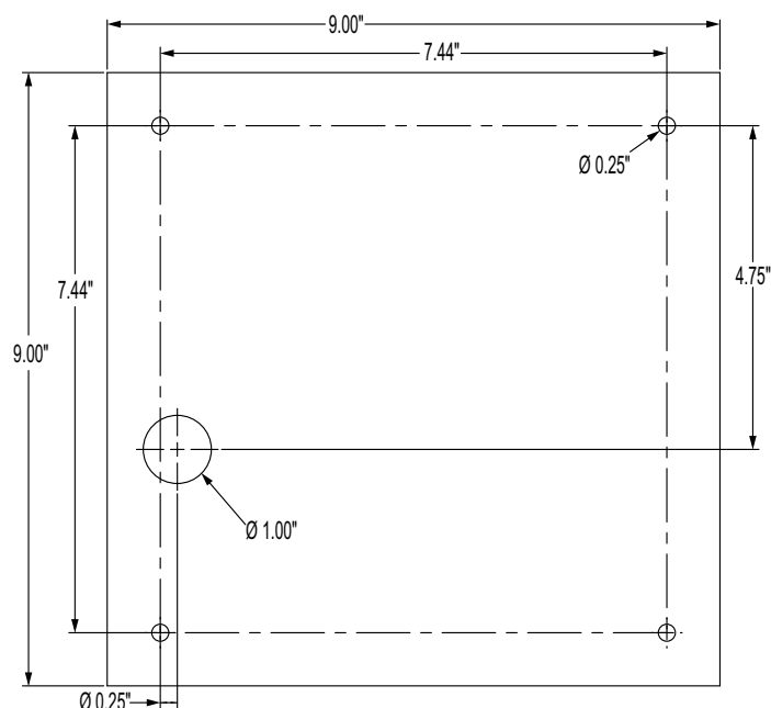
Figura 2-15. Dimensioni della versione da 7" con montaggio a pannello (con tastiera)
