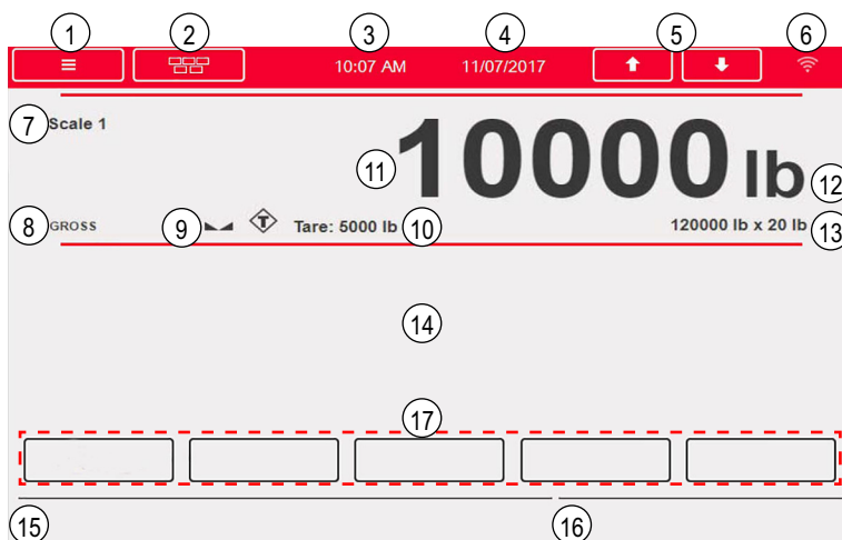
Figura 1-1. Schermo del display della modalità di pesatura
