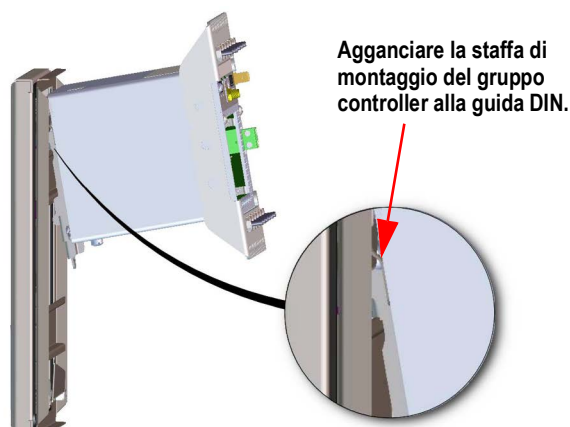
Figura 2-20. Aggancio della piastra di montaggio alla guida DIN
