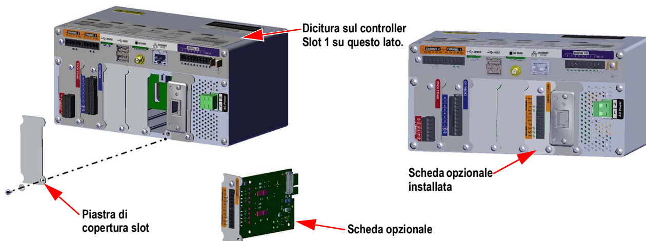
Figura 2-24. Installazione della scheda opzionale
