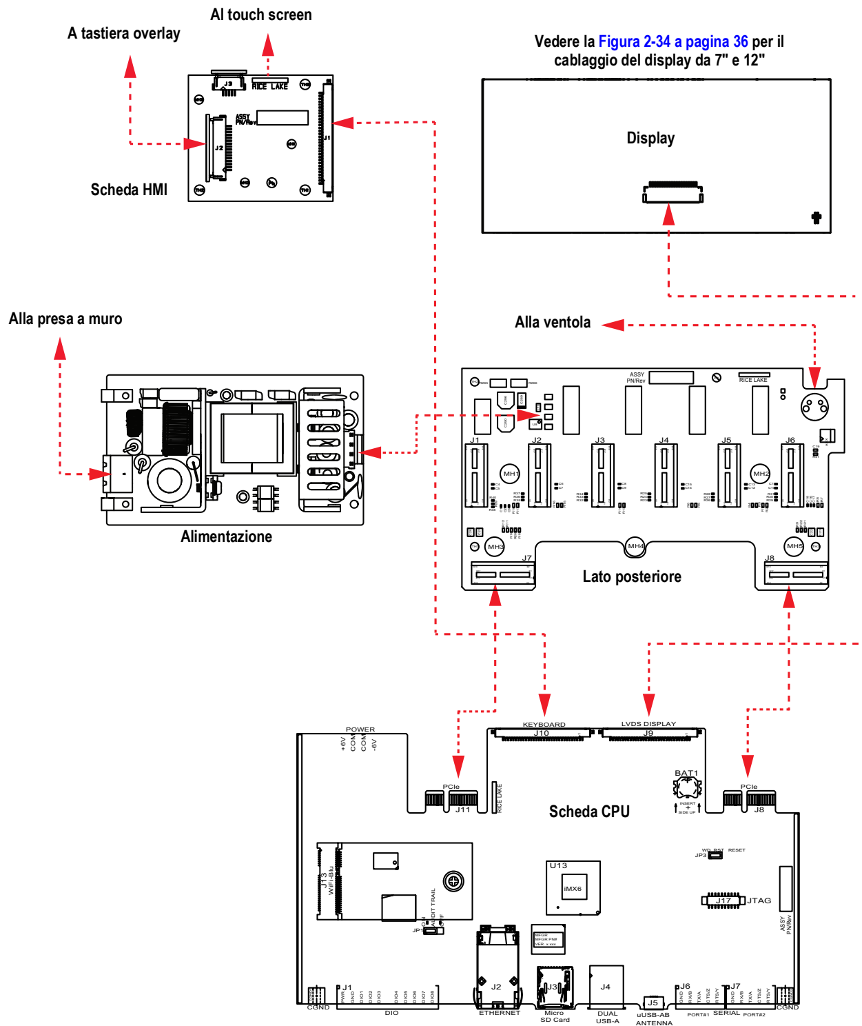
Figura 2-33. Schema di cablaggio
