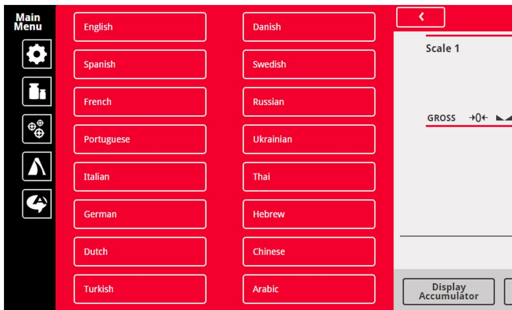
Figura 1-6. Lingue selezionabili
