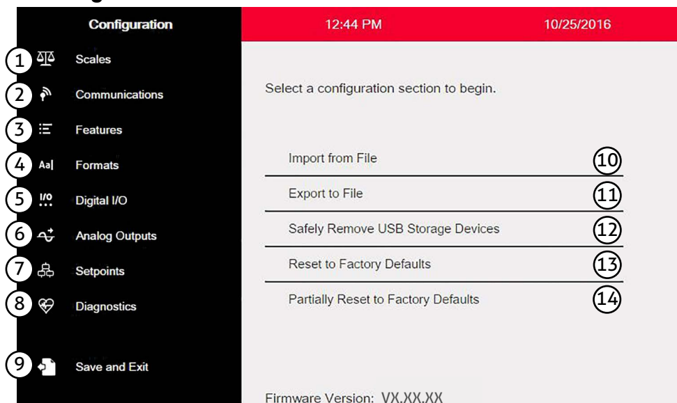
Figura 3-4. Menu di configurazione
