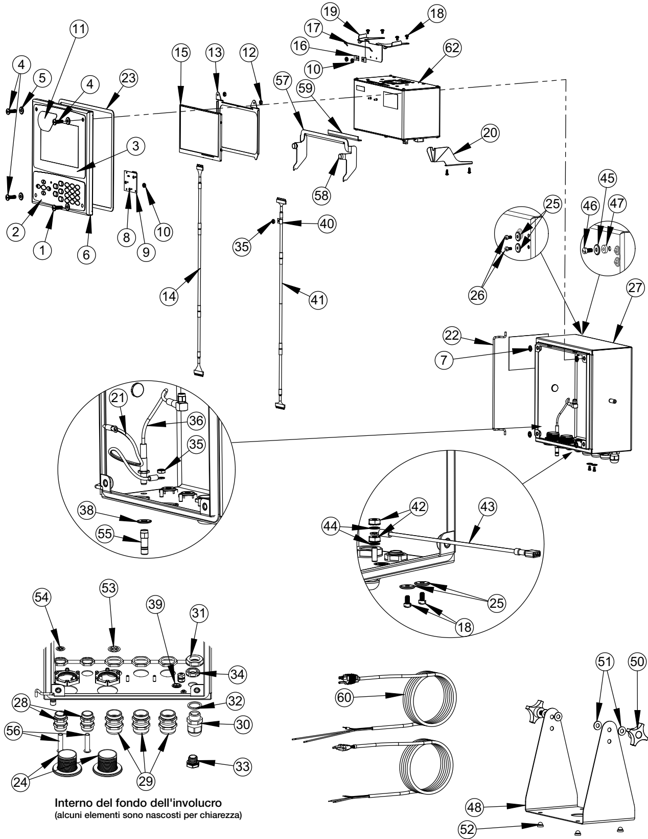
Figura 2-40. Componenti per la riparazione dell'indicatore con montaggio universale
