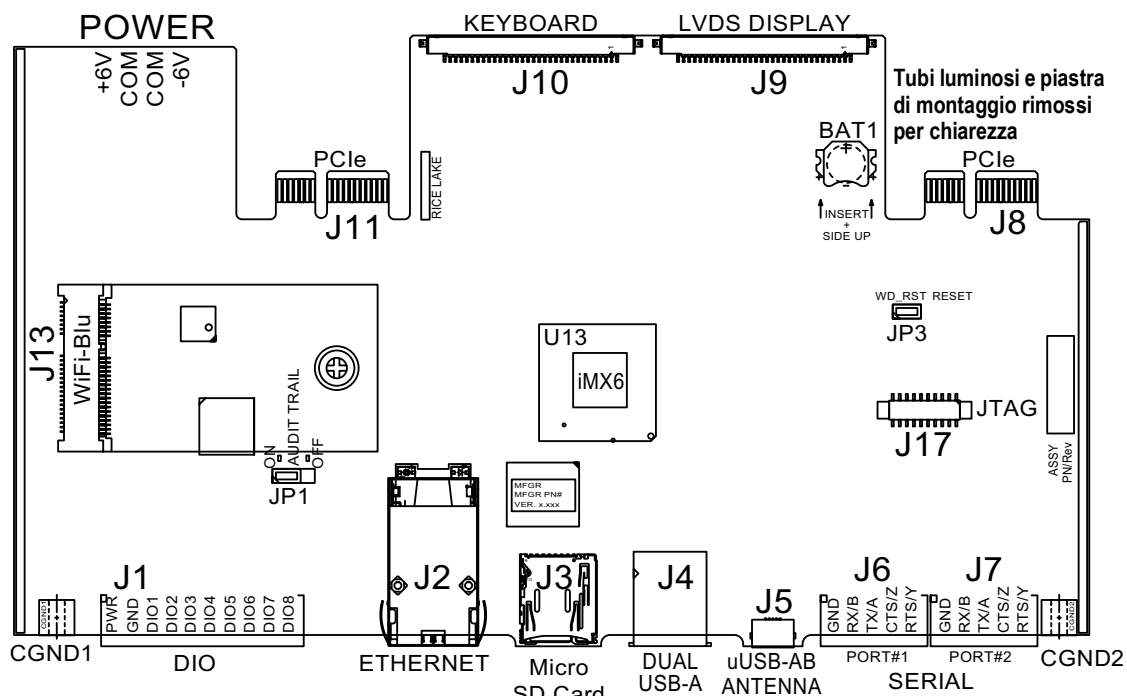
Figura 2-32. Scheda CPU (vista dall'alto)
