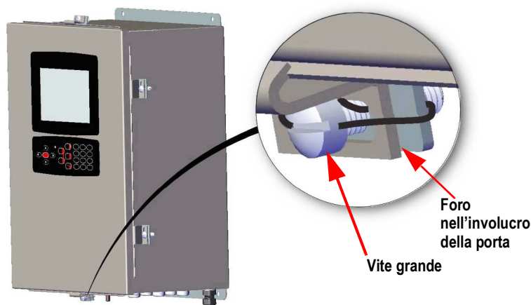
Figura 2-13. Sigillatura della porta anteriore
