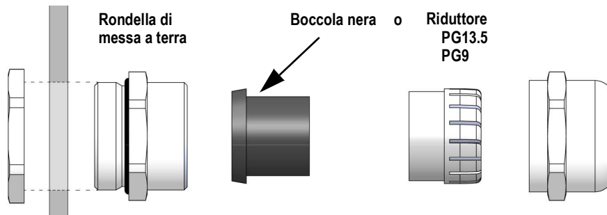
Figura 2-26. Pressacavo con riduttore
