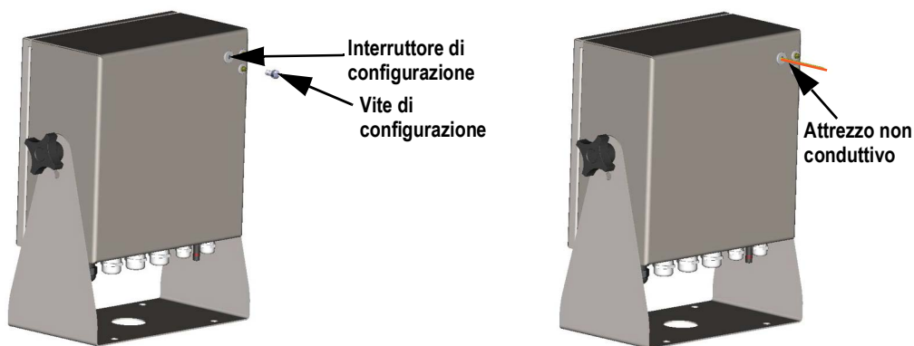
Figura 3-1. Posizione dell'interruttore di configurazione (involucro universale)
