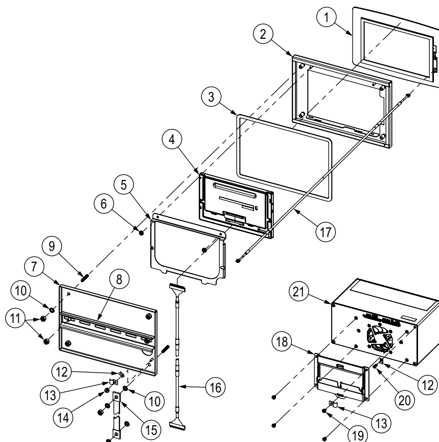
Figura 2-44. Componenti per la riparazione dell'indicatore da 7" con montaggio a pannello solo touch
