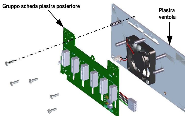
Figura 2-38. Rimozione del gruppo scheda piastra posteriore
