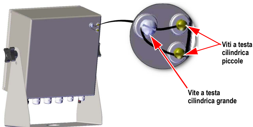
Figura 2-6. Sigillare l'interruttore di configurazione (supporto universale)
