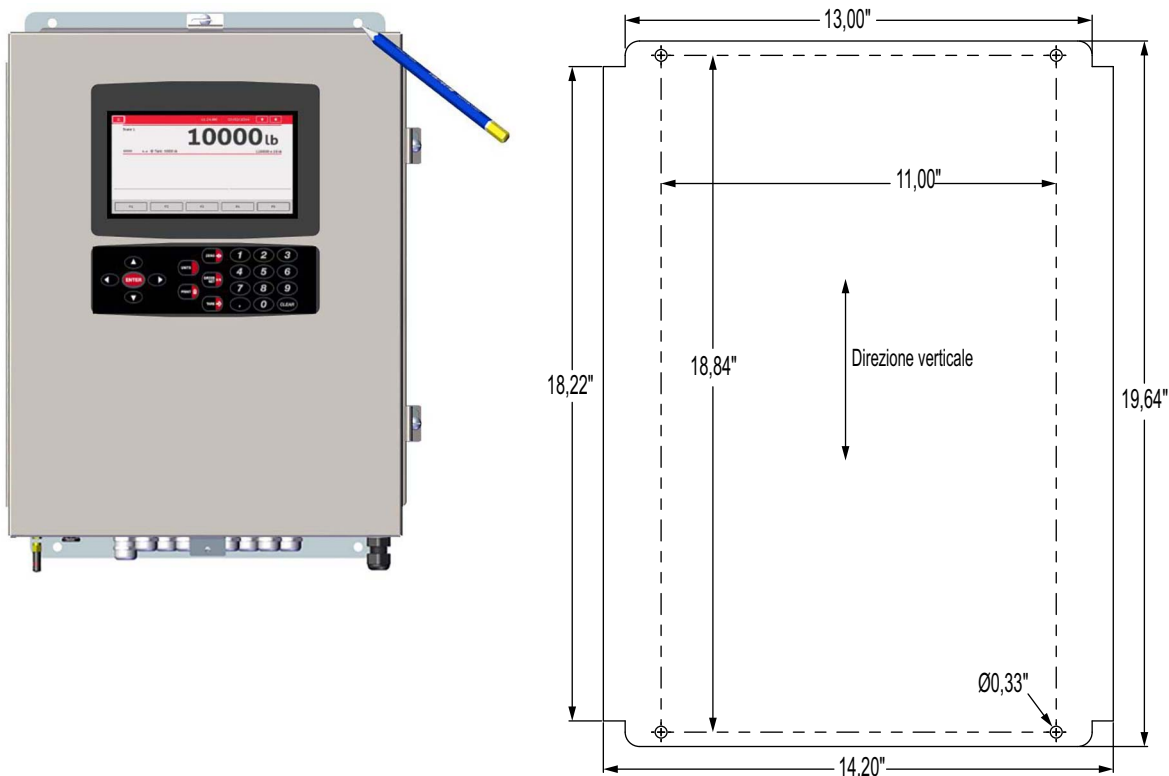
Figura 2-8. Montaggio a parete
