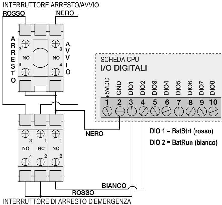
Figura 10-14. Esempio di schema di cablaggio dell'interruttore di batch
