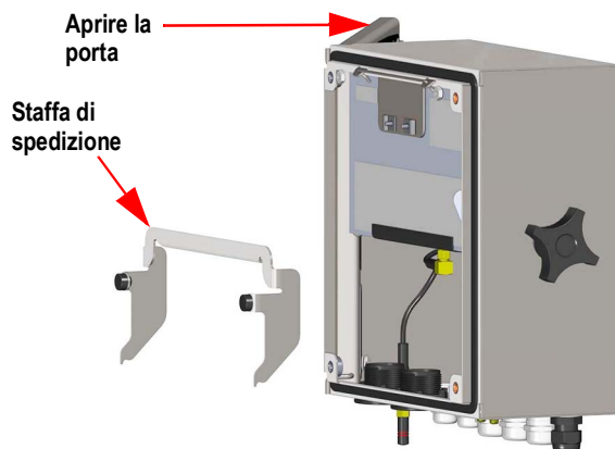
Figura 2-2. Rimuovere la staffa di spedizione
