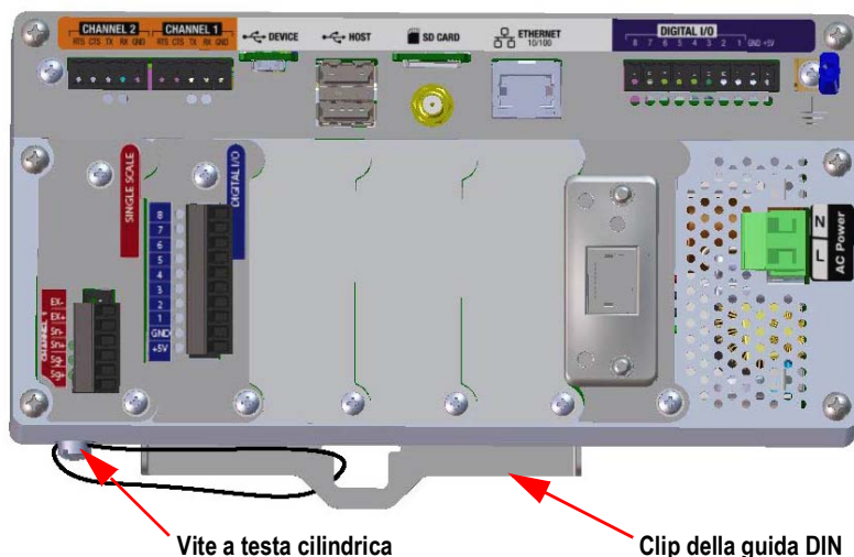
Figura 2-12. Sigillatura dell'interruttore di configurazione
