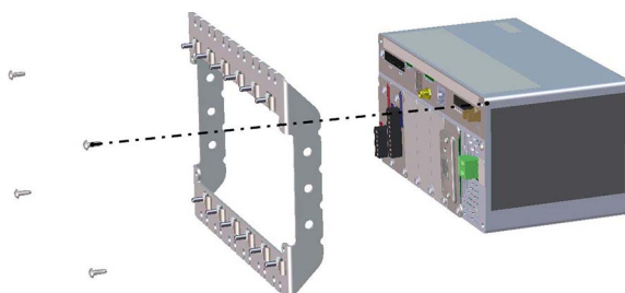
Figura 2-18. Installazione della sbarra di messa a terra
