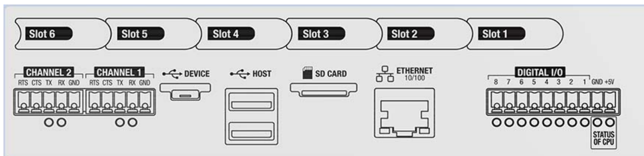
Figura 2-23. Diciture sulla parte superiore del gruppo controller
