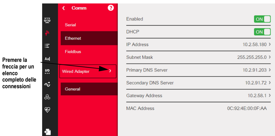
Figura 5-3. Schermata Ethernet
