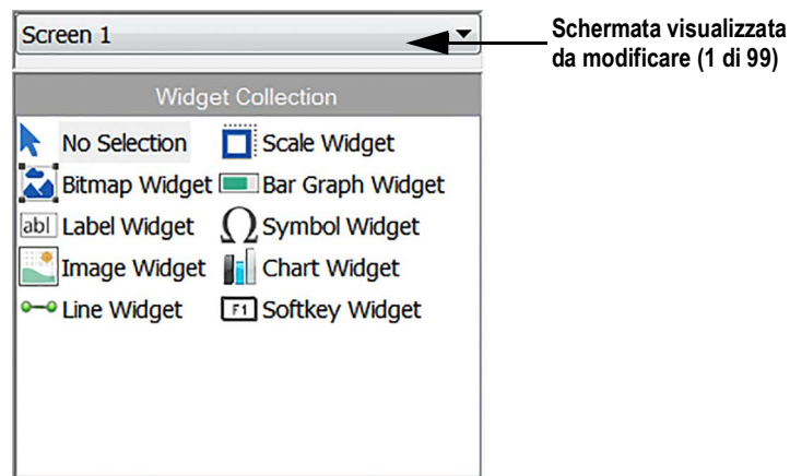
Figura 14-1. Schermata Widget
