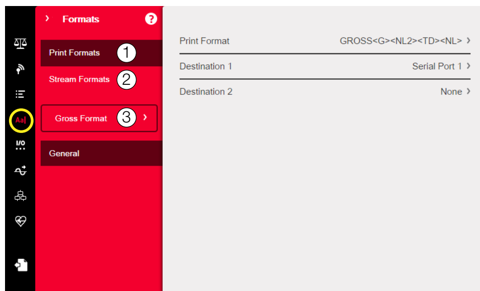
Figura 7-1. Menu Formats
