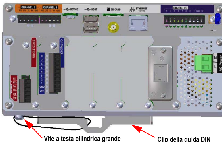
Figura 2-22. Sigillare l'interruttore di configurazione (involucro con montaggio a pannello)
