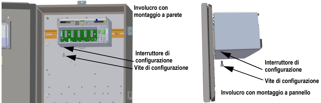
Figura 3-2. Posizioni dell'interruttore di configurazione (involucri con montaggio a pannello/parete)
