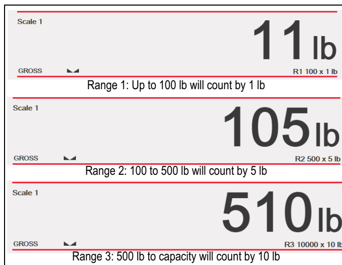
Figura 4-4. Esempio di Multi-Range
