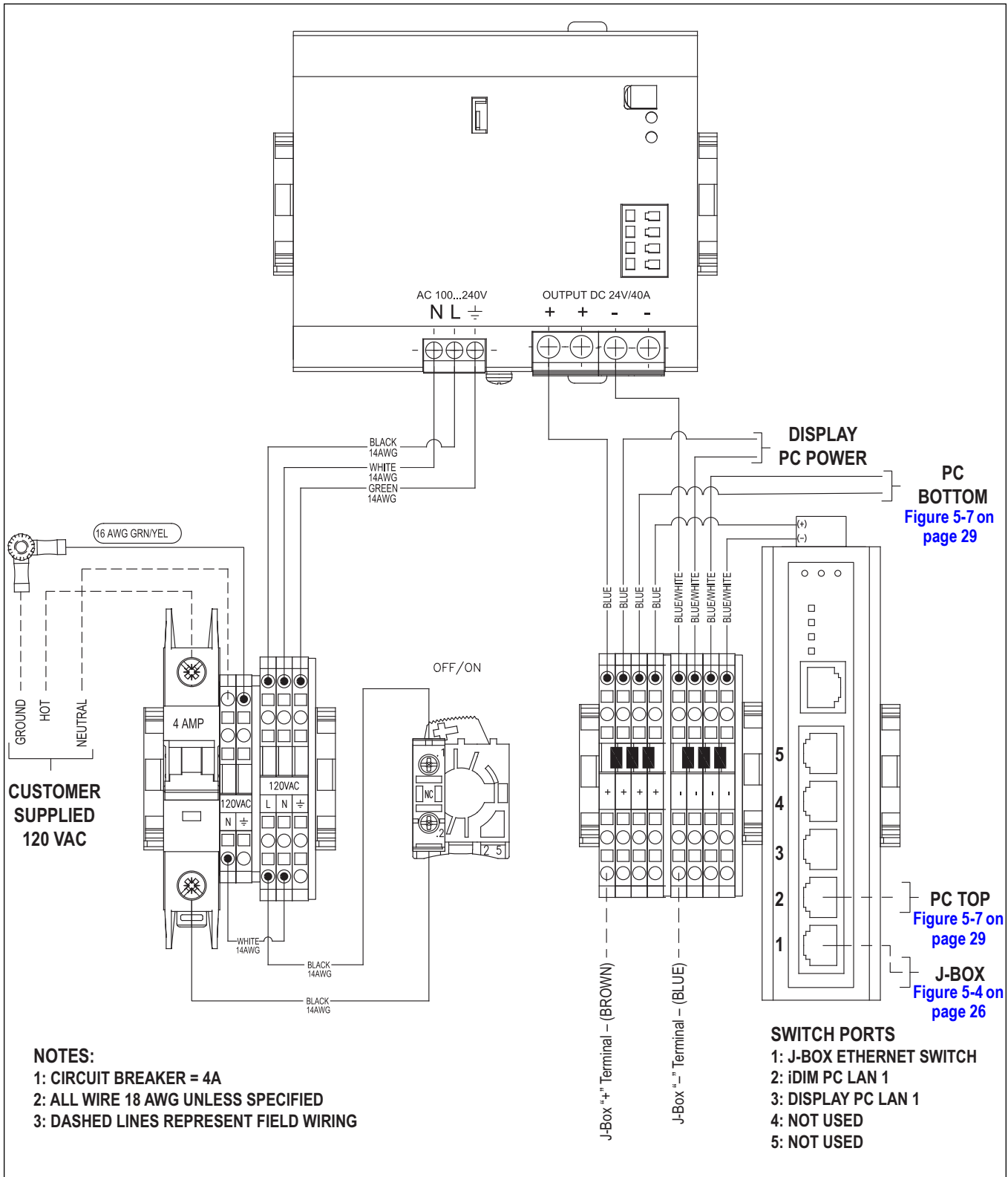
Figure 5-6. Kiosk Wiring
